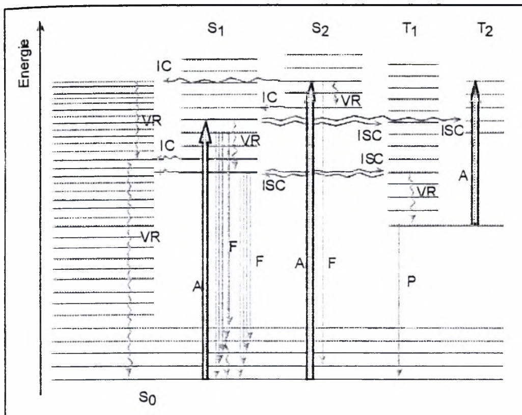
Εικόνα 2-1. Απλοποιημένο διάγραμμα Jablonki (Συντμ.: A=απορρόφηση, διέγερση , F =φθορισμός , P = φωσφορισμός , VR= ταλαντώσεις , IC= εσωτερική μετατροπή , ISC= εσωτερικοί συνδιασμοί μετατροπών).
