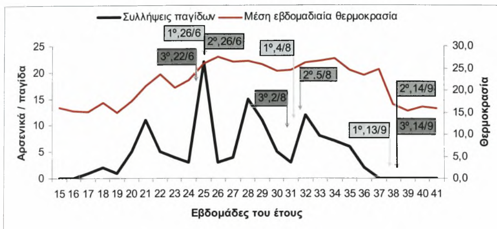
Σχήμα 5.1. Συλλήψεις αρσενικών ατόμων C. rotonella σε φερομονικές παγίδες τα έτη, 2002 (a), 2003 (b), 2005 (c), 2006 (d), 2007 (e), 2008 (f) και απεικόνιση των αποτελεσμάτων των τριών μοντέλων στην Αγιά Λάρισα.
