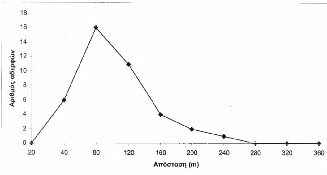
Σχήμα 8.4. Ο αριθμός αδερφών σε σχέση με την απόσταση.
