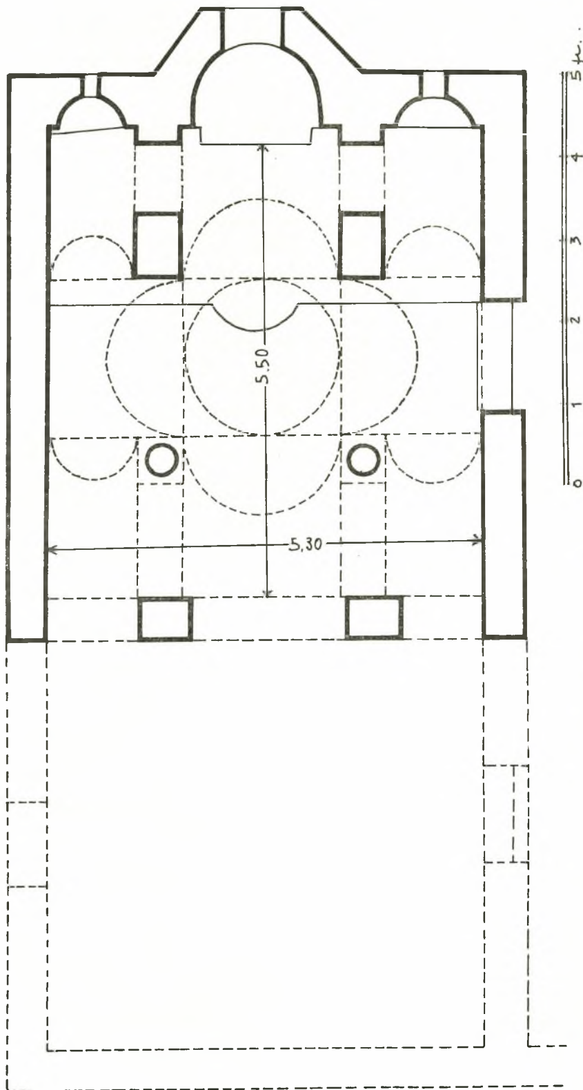
Εικ. 1. Άγιος Νικόλαος Μεγούλας. Κάτοψις.
