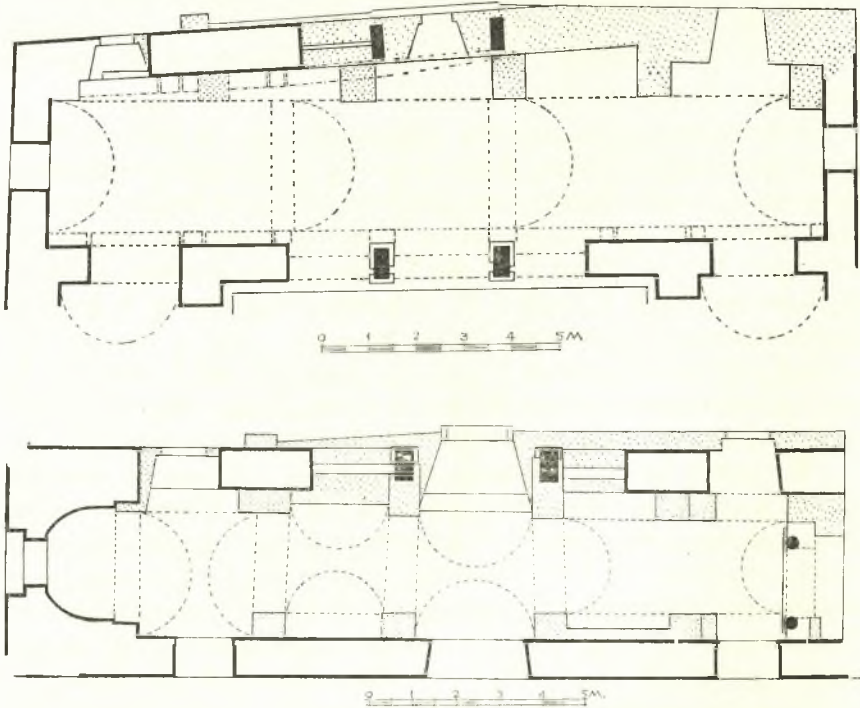
Εἰκ. 3 Κάτω: ὀριζοντία τομὴ τοῦ ἰσογείου τοῦ νάρθηκος ἄνω τῆς βορείου κόγχης. Ἄνω: ὀριζοντία τομὴ τοῦ γυναικωνίτου τοῦ νάρθηκος. Ἀμφότεραι ἐμφαίνουσι τὴν κατάστασιν πρὸ τῆς κατεδαφίσεως τῶν μεταγενεστέρων προσθηκῶν.
