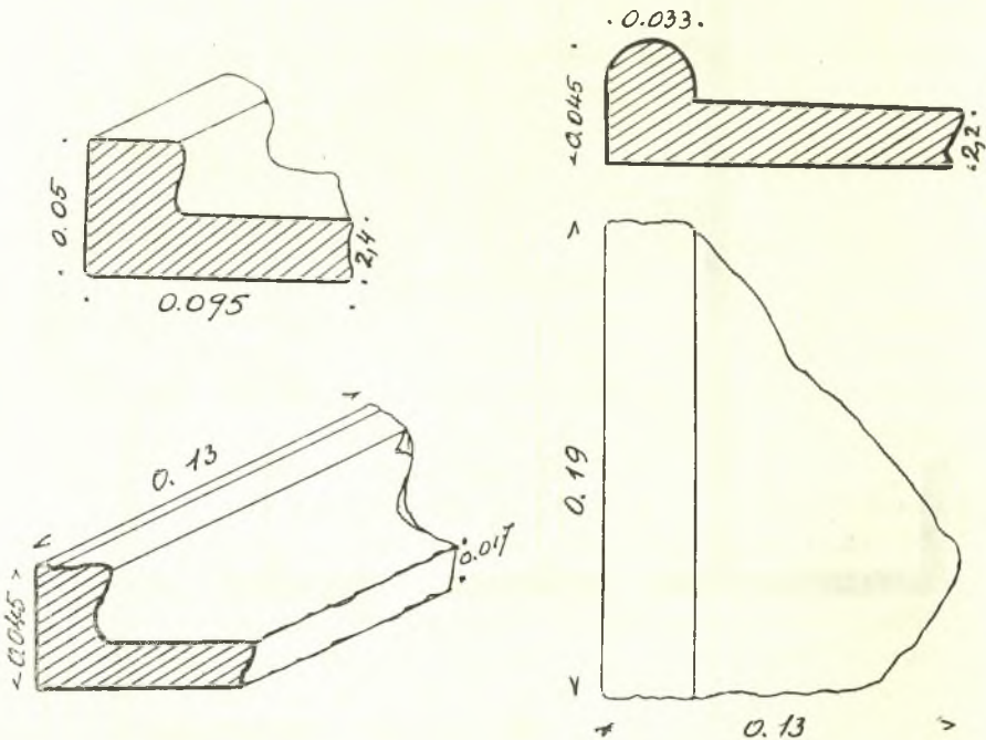
Εἰκ. 2. Στρωτῆρες πήλινοι κέραμοι ἐκ τῆς στέγης.
