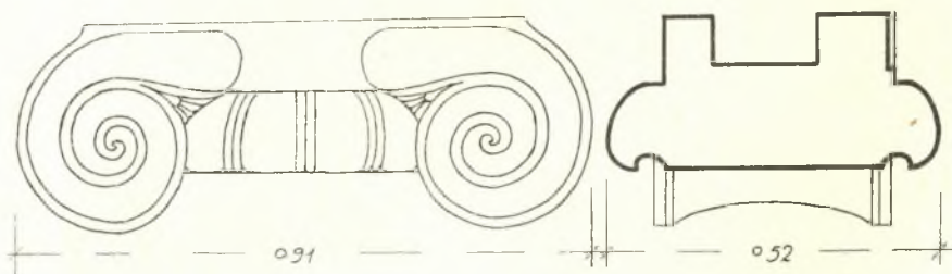
Εἰκ. 9. Πρόσοψις καὶ τομὴ τοῦ ἀρχαίου ἰωνικοῦ κιονοκράνου, ἐφ' οὗ ἡ ἐπιγραφή τοῦ Ἀρχιλόχου.
