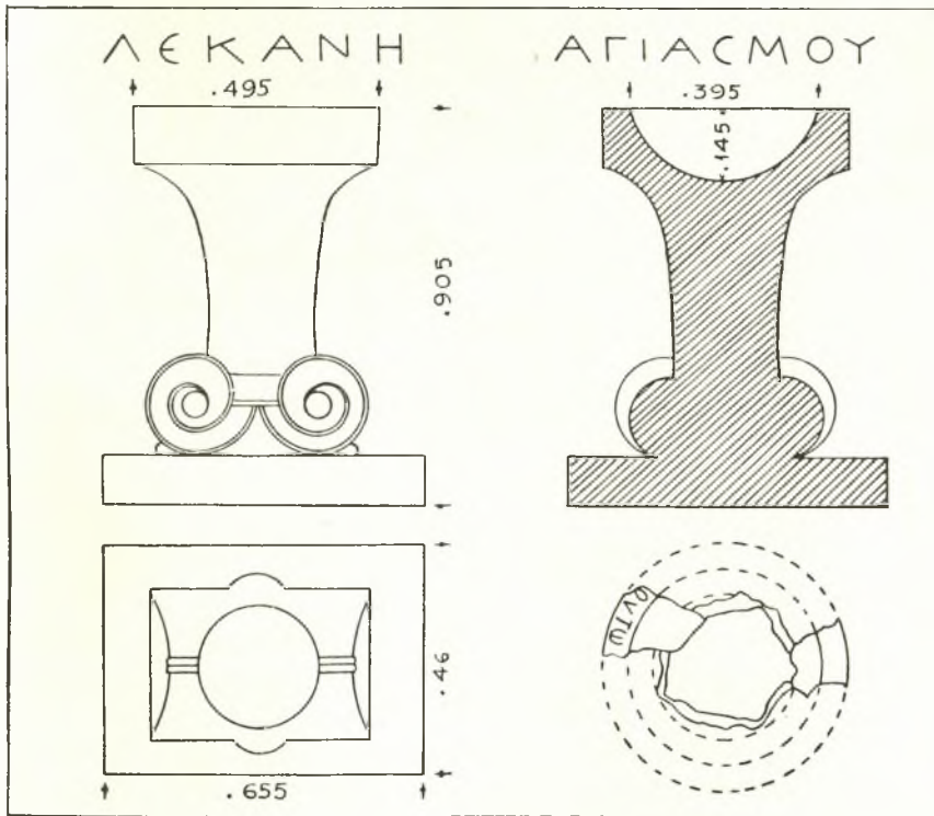
Εἰκ. 8. Λεκάνη ἁγιασμοῦ εὑρεθεῖσα κατὰ χώραν ἐντὸς τοῦ νάρθηκος καὶ εὐθὺς παρὰ τὴν βασιλείον πύλην.
