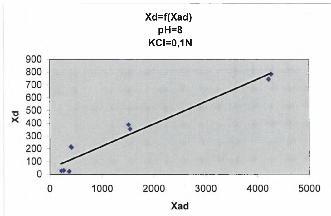
Διάγραμμα 3.1-5: Η εκρόφιση του καδμίου X_d (μg Cd/g γκαϊτίτη) σε συνάρτηση με την προσρόφιση του καδμίου X_{ad} (μg Cd/g γκαϊτίτη) σε pH=8 και ηλεκτρολύτη KCl 0,1N.
