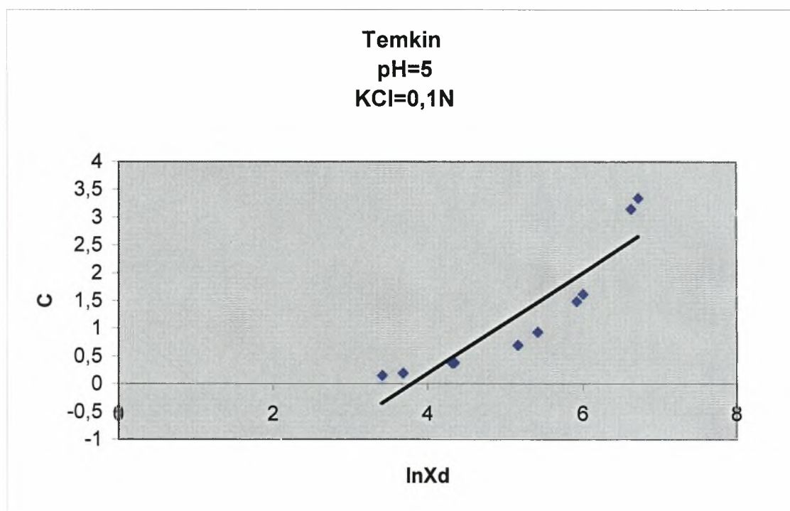
Διάγραμμα 3.4-2: Η συγκέντρωση ισορροπίας (C mg/L) σε συνάρτηση με την ln του ποσού που εκροφάται σε pH=5 και παρουσία ηλεκτρολύτη KCl=0,1N.
