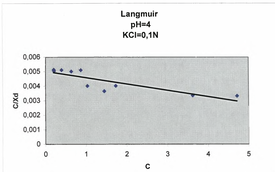
Διάγραμμα 3.2-1: Ο λόγος της συγκέντρωσης ισορροπίας ( C mg/L) προς το ποσό της ουσίας που εκροφάται ( X_d mg/kg) σε συνάρτηση με τη συγκέντρωση ισορροπίας σε pH=4 και παρουσία ηλεκτρολύτη KCl=0,1N.
