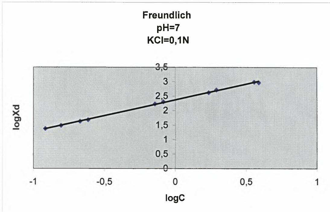
Διάγραμμα 3.3-4: Ο λογάριθμος του ποσού που εκροφάται σε συνάρτηση με τον λογάριθμο της συγκέντρωσης ισορροπίας σε pH=7 και παρουσία ηλεκτρολύτη KCl=0,1N.
