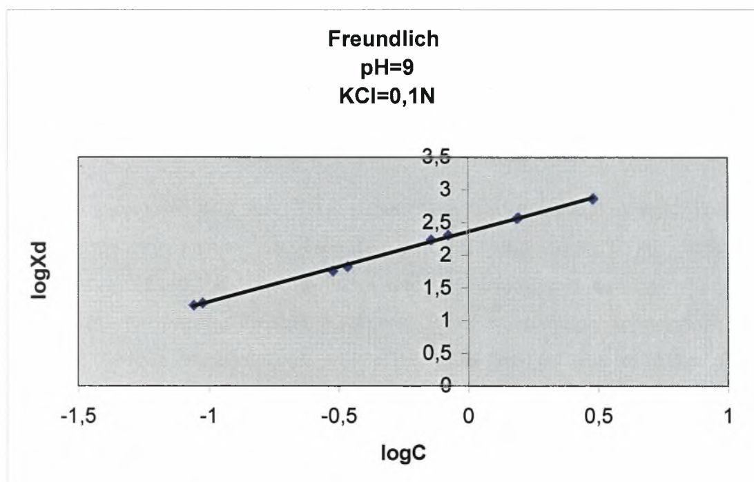
Διάγραμμα 3.3-6: Ο λογάριθμος του ποσού που εκροφάται σε συνάρτηση με τον λογάριθμο της συγκέντρωσης ισορροπίας σε pH=9 και παρουσία ηλεκτρολύτη KCl=0,1N.
