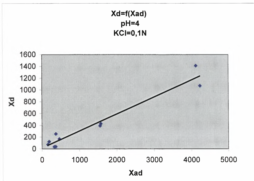
Διάγραμμα 3.1-1: Η εκρόφιση του καδμίου X_d (μg Cd/g γκαϊτίτη) σε συνάρτηση με την προσρόφιση του καδμίου X_{ad} (μg Cd/g γκαϊτίτη) σε pH=4 και ηλεκτρολύτη KCl 0,1N
