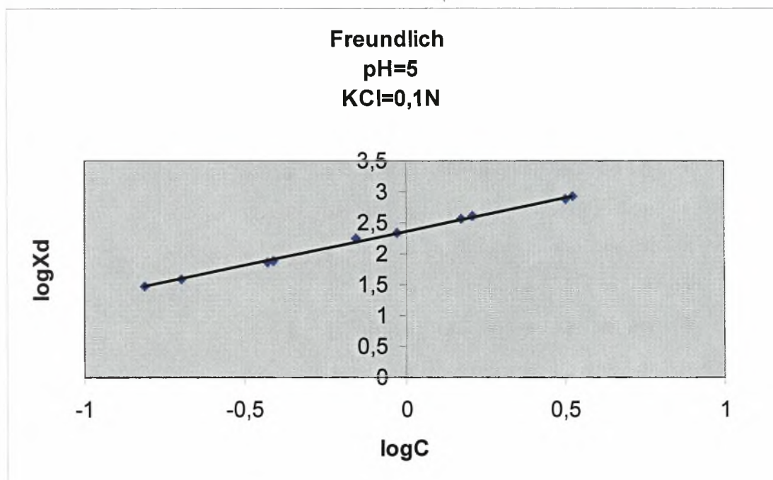
Διάγραμμα 3.3-2: Ο λογάριθμος του ποσού που εκροφάται σε συνάρτηση με τον λογάριθμο της συγκέντρωσης ισορροπίας σε pH=5 και παρουσία ηλεκτρολύτη KCl=0,1N.
