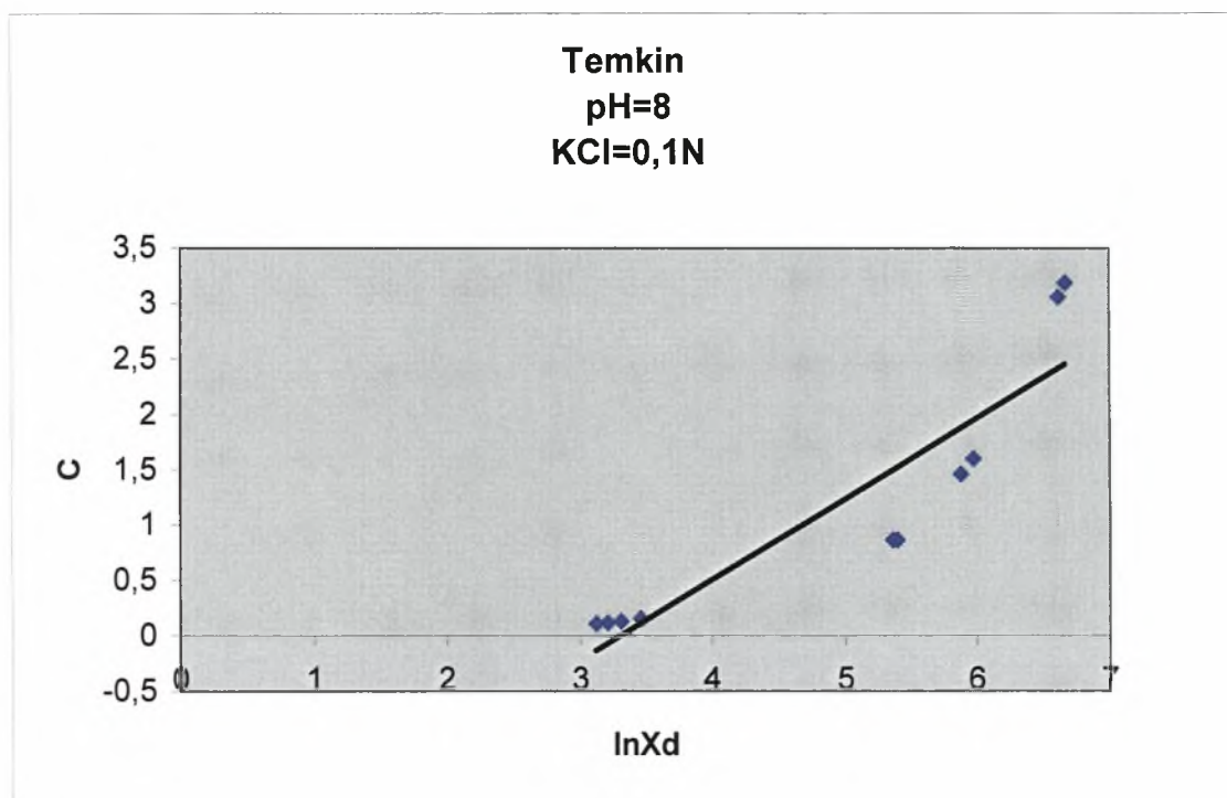
Διάγραμμα 3.4-5: Η συγκέντρωση ισορροπίας ( C mg/L) σε συνάρτηση με την \ln του ποσού που εκροφάται σε \text{pH}=8 και παρουσία ηλεκτρολύτη \text{KCl}=0,1\text{N} .
