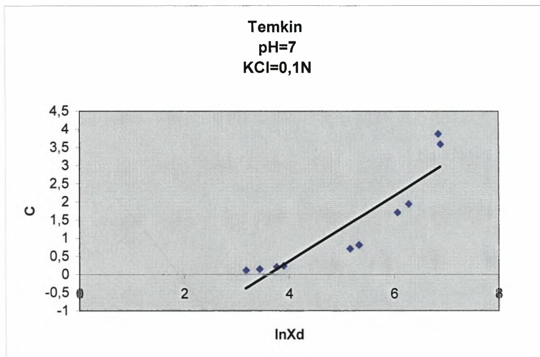
Διάγραμμα 3.4-4: Η συγκέντρωση ισορροπίας ( C mg/L) σε συνάρτηση με την \ln του ποσού που εκροφάται σε \text{pH}=7 και παρουσία ηλεκτρολύτη \text{KCl}=0,1\text{N} .
