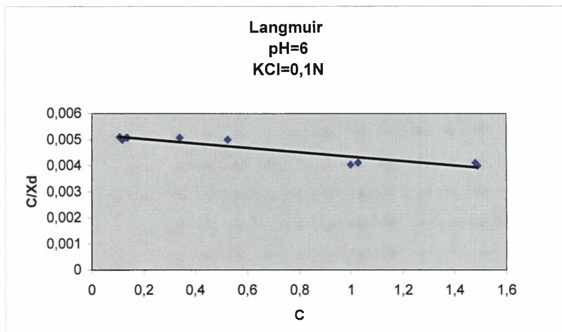
Διάγραμμα 3.2-3: Ο λόγος της συγκέντρωσης ισορροπίας ( C mg/L) προς το ποσό της ουσίας που εκροφάται ( X_d mg/kg) σε συνάρτηση με τη συγκέντρωση ισορροπίας σε pH=6 και παρουσία ηλεκτρολύτη KCl=0,1N.
