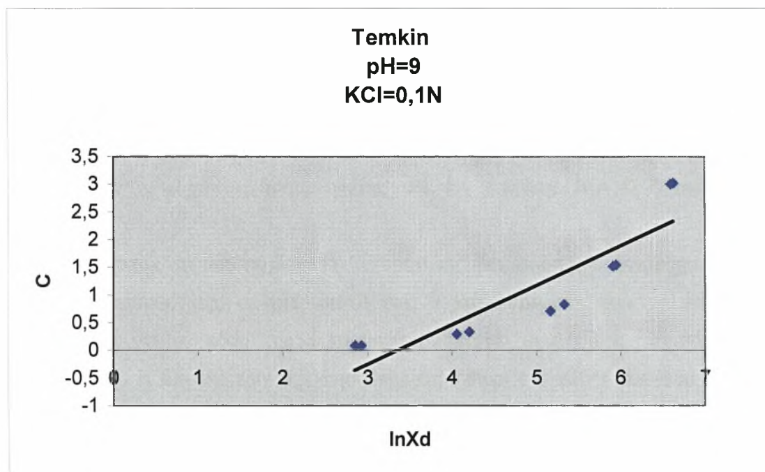
Διάγραμμα 3.4-6: Η συγκέντρωση ισορροπίας ( C mg/L) σε συνάρτηση με την \ln του ποσού που εκροφάται σε \text{pH}=9 και παρουσία ηλεκτρολύτη \text{KCl}=0,1\text{N} .
