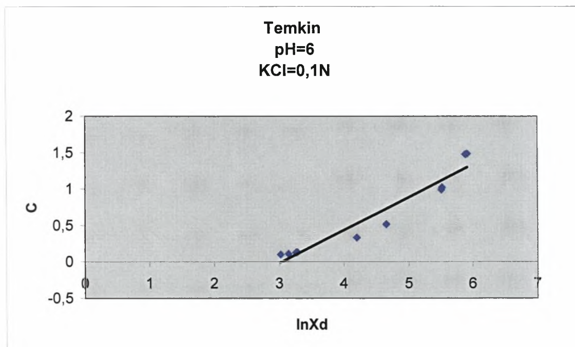
Διάγραμμα 3.4-3: Η συγκέντρωση ισορροπίας (C mg/L) σε συνάρτηση με την ln του ποσού που εκροφάται σε pH=6 και παρουσία ηλεκτρολύτη KCl=0,1N.
