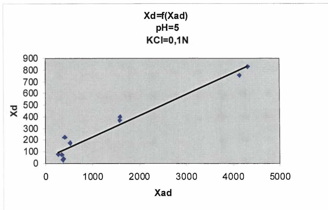
Διάγραμμα 3.1-2: Η εκρόφιση του καδμίου X_d (μg Cd/g γκαίτιτη) σε συνάρτηση με την προσρόφιση του καδμίου X_{ad} (μg Cd/g γκαίτιτη) σε pH=5 και ηλεκτρολύτη KCl 0,1N
