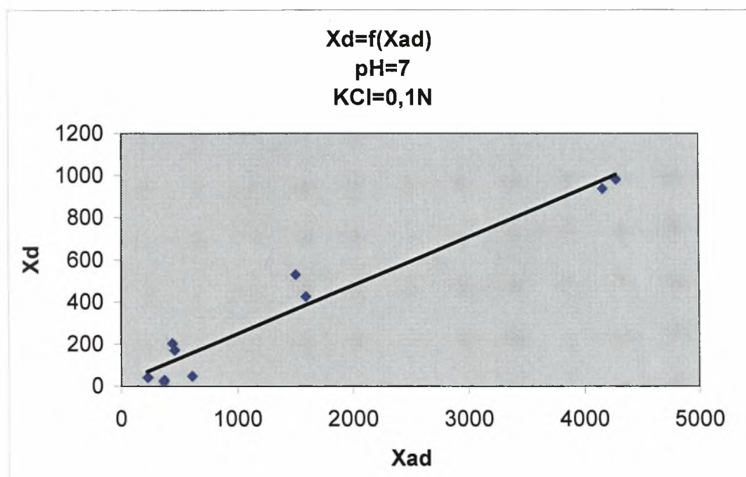
Διάγραμμα 3.1-4: Η εκρόφιση του καδμίου X_d ( \mu\text{g Cd/g} γκαϊτίτη) σε συνάρτηση με την προσρόφιση του καδμίου X_{ad} ( \mu\text{g Cd/g} γκαϊτίτη) σε pH=7 και ηλεκτρολύτη KCl 0,1N.
