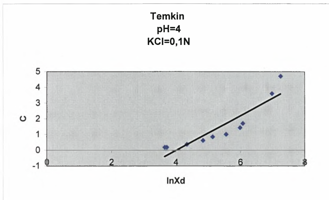
Διάγραμμα 3.4-1: Η συγκέντρωση ισορροπίας (C mg/L) σε συνάρτηση με την ln του ποσού που εκροφάται σε pH=4 και παρουσία ηλεκτρολύτη KCl=0,1N.
