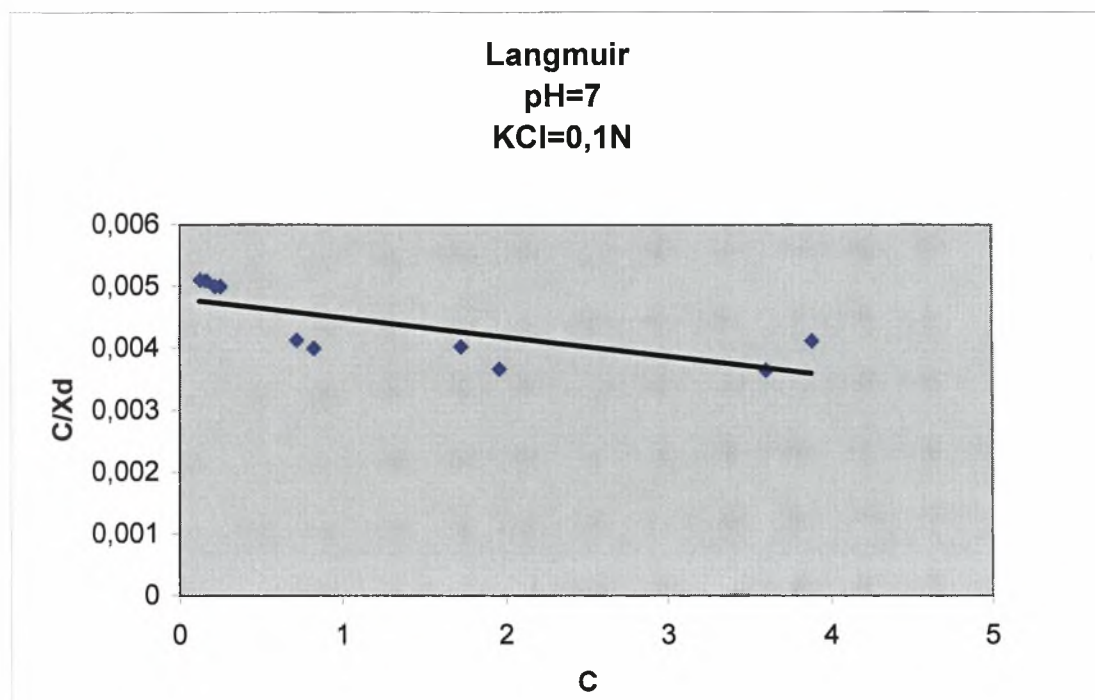
Διάγραμμα 3.2-4: Ο λόγος της συγκέντρωσης ισορροπίας (C mg/L) προς το ποσό της ουσίας που εκροφάται (Xd mg/kg) σε συνάρτηση με τη συγκέντρωση ισορροπίας σε pH=7 και παρουσία ηλεκτρολύτη KCl=0,1N.
