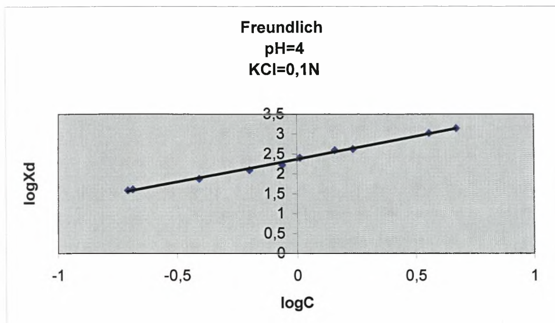
Διάγραμμα 3.3-1: Ο λογάριθμος του ποσού που εκροφάται σε συνάρτηση με τον λογάριθμο της συγκέντρωσης ισορροπίας σε pH=4 και παρουσία ηλεκτρολύτη KCl=0,1N.
