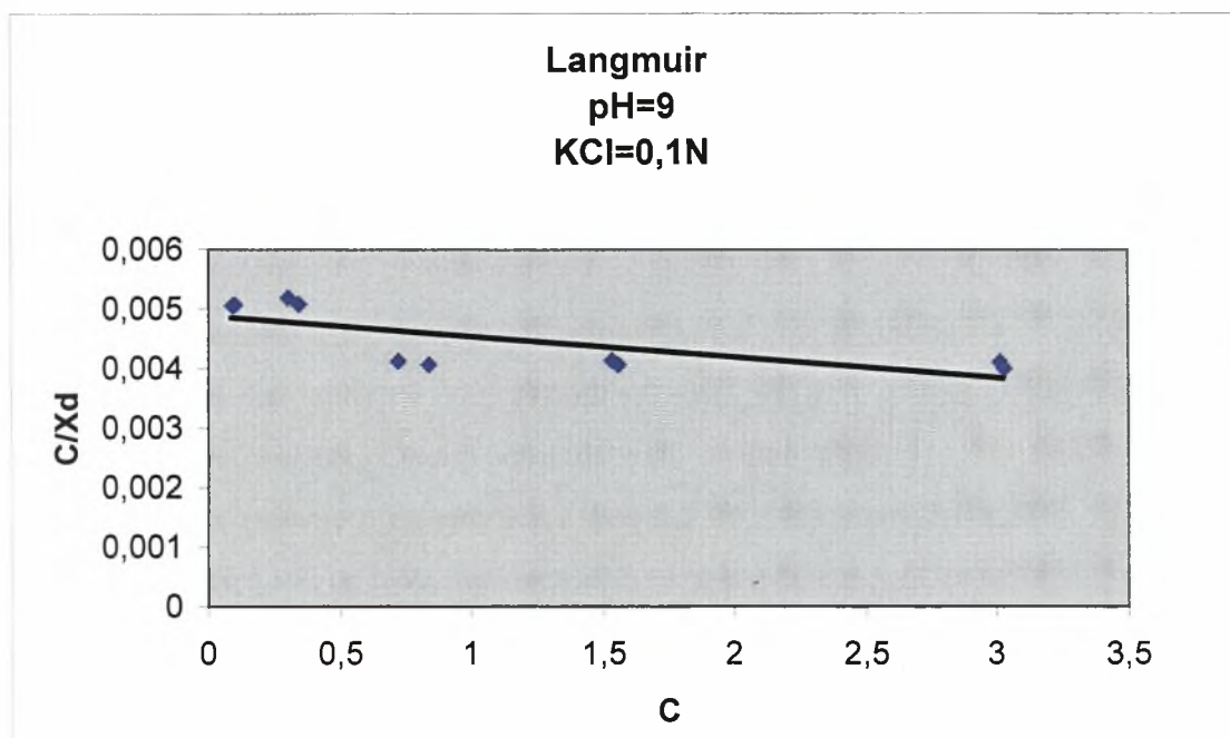
Διάγραμμα 3.2-6: Ο λόγος της συγκέντρωσης ισορροπίας ( C mg/L) προς το ποσό της ουσίας που εκροφάται ( X_d mg/kg) σε συνάρτηση με τη συγκέντρωση ισορροπίας σε pH=9 και παρουσία ηλεκτρολύτη KCl=0,1N.
