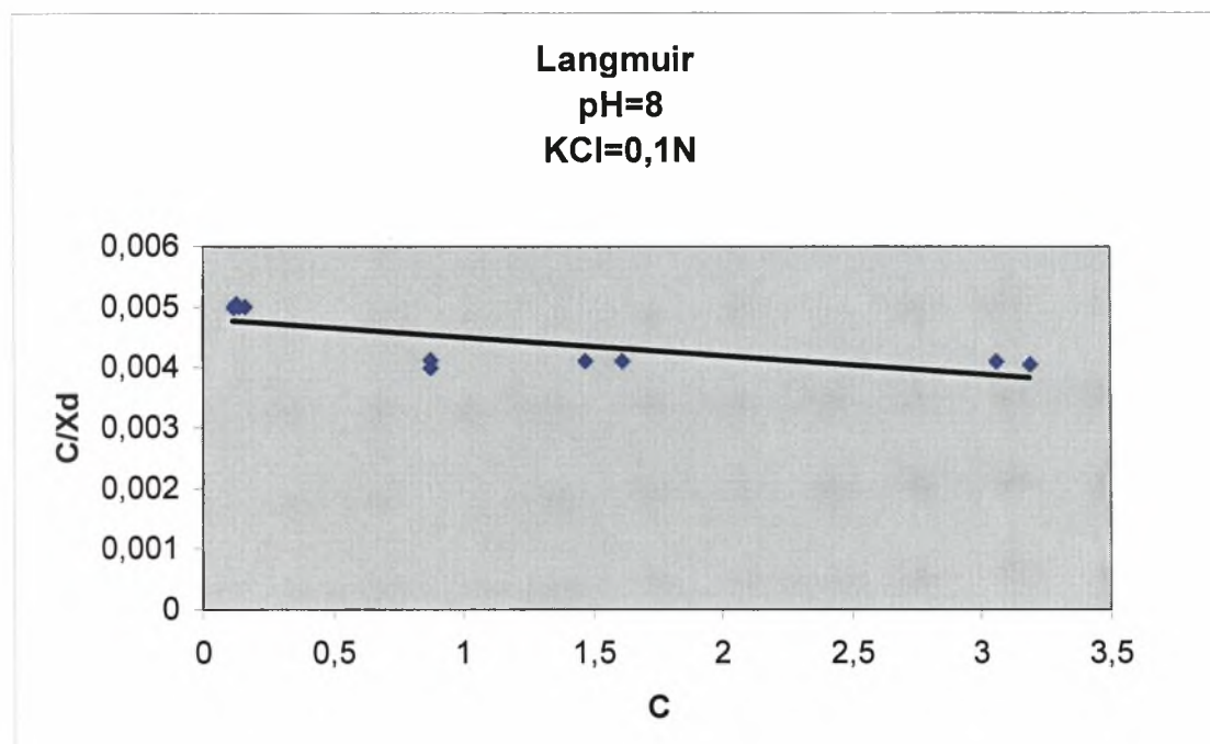
Διάγραμμα 3.2-5: Ο λόγος της συγκέντρωσης ισορροπίας (C mg/L) προς το ποσό της ουσίας που εκροφάται (Xd mg/kg) σε συνάρτηση με τη συγκέντρωση ισορροπίας σε pH=8 και παρουσία ηλεκτρολύτη KCl=0,1N.
