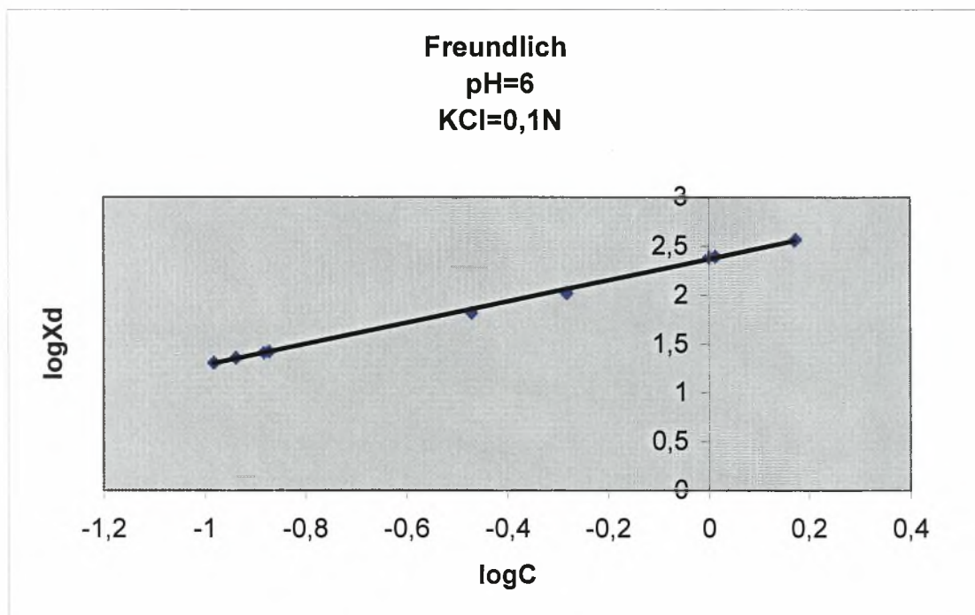
Διάγραμμα 3.3-3: Ο λογάριθμος του ποσού που εκροφάται σε συνάρτηση με τον λογάριθμο της συγκέντρωσης ισορροπίας σε pH=6 και παρουσία ηλεκτρολύτη KCl=0,1N.
