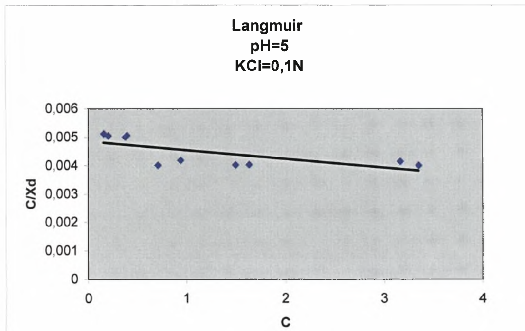
Διάγραμμα 3.2-2: Ο λόγος της συγκέντρωσης ισορροπίας ( C mg/L) προς το ποσό της ουσίας που εκροφάται ( X_d mg/kg) σε συνάρτηση με τη συγκέντρωση ισορροπίας σε pH=5 και παρουσία ηλεκτρολύτη KCl=0,1N .
