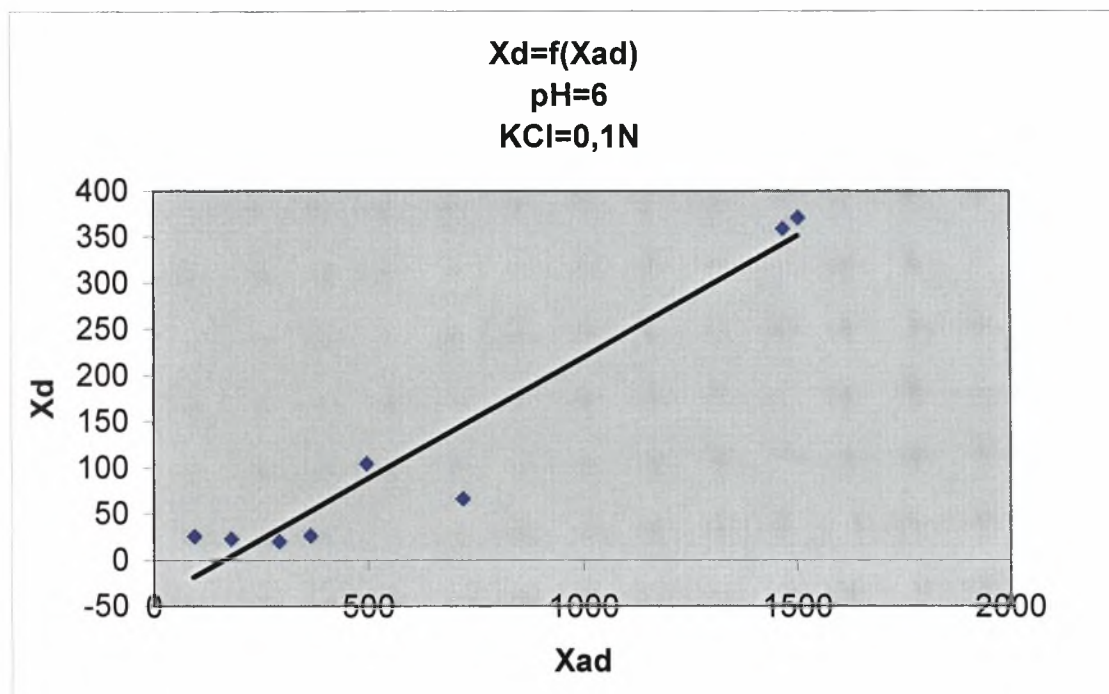
Διάγραμμα 3.1-3: Η εκρόφιση του καδμίου X_d ( \mu\text{g Cd/g} γκαϊτίτη) σε συνάρτηση με την προσρόφιση του καδμίου X_{ad} ( \mu\text{g Cd/g} γκαϊτίτη) σε pH=6 και ηλεκτρολύτη KCl 0,1N.
