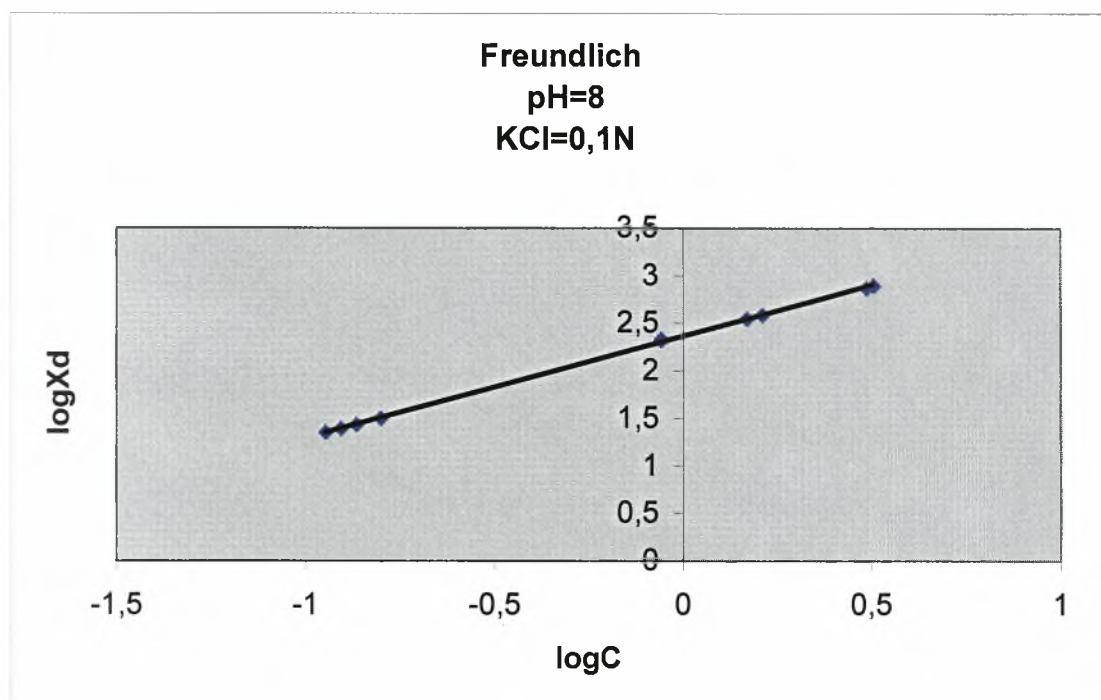
Διάγραμμα 3.3-5: Ο λογάριθμος του ποσού που εκροφάται σε συνάρτηση με τον λογάριθμο της συγκέντρωσης ισορροπίας σε pH=8 και παρουσία ηλεκτρολύτη KCl=0,1N.
