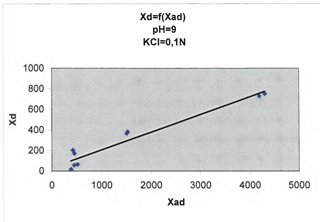
Διάγραμμα 3.1-6: Η εκρόφιση του καδμίου X_d ( \mu\text{g Cd/g} γκαιοίτη) σε συνάρτηση με την προσρόφιση του καδμίου X_{ad} ( \mu\text{g Cd/g} γκαιοίτη) σε pH=9 και ηλεκτρολύτη KCl 0,1N.
