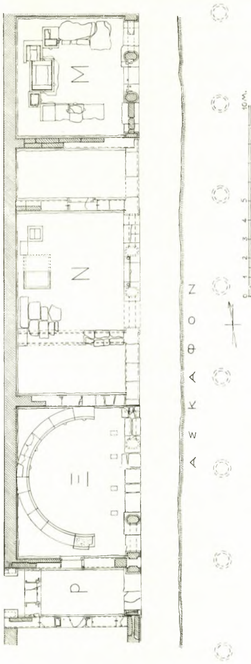
Εικ. 2. Κάτοψις τῶν κατὰ τὸ 1963 ἀποκαλυφθέντων διαμερισμάτων τῆς δυτικῆς πλευρᾶς τοῦ τετραστύλου συγκροτήματος τῆς «Λαγοῦρας».
