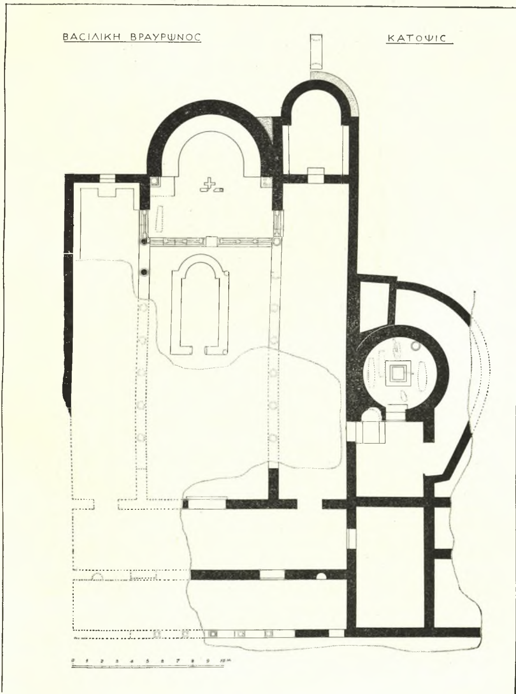
Εικ. 3. Κάτοψις τῆς ἀνασκαφείσης παρά τὴν Βραυρῶνα βασιλικῆς.
