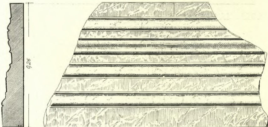
Εἰκ. 9. Τμῆμα τοῦ μαρμαρίνου τοιχοβάτου (τομὴ καὶ ὀρθὴ προβολή).
