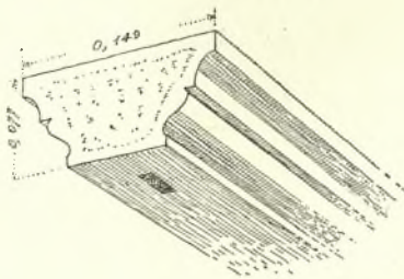
Εἰκ. 19. Στέψις τῶν θωρακίων.
