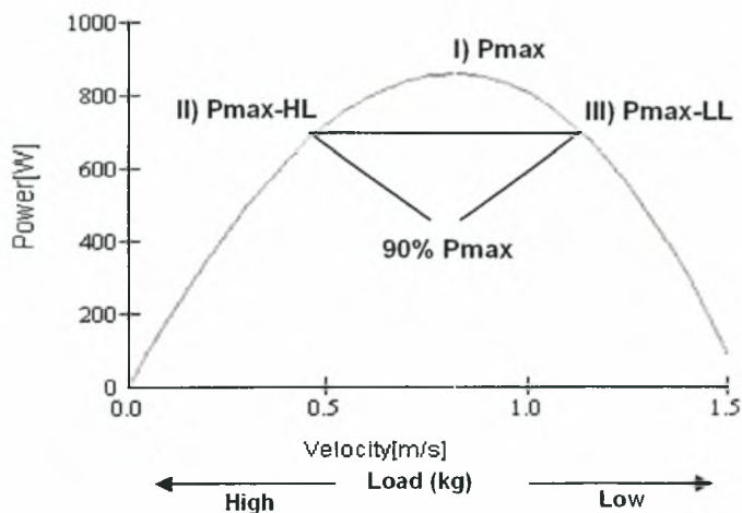
Σχήμα 3.2: Η ταχοδυναμική καμπύλη, από την οποία προσδιορίζονταν οι τρεις πειραματικές συνθήκες βάσει της παραγόμενης ισχύος
