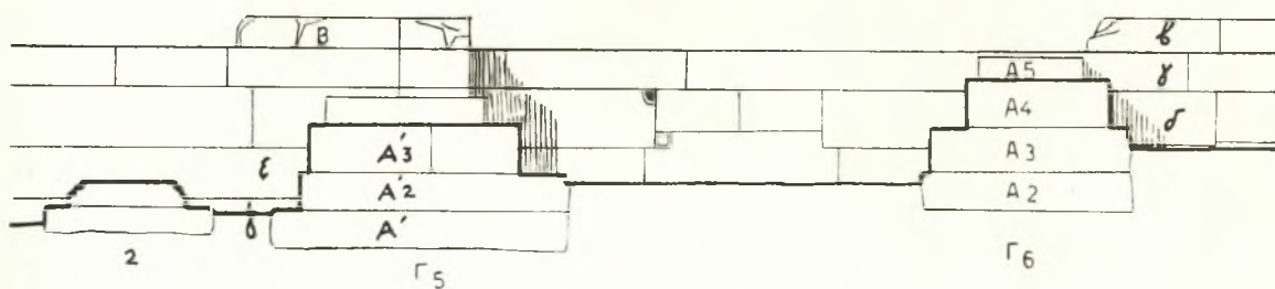
Εἰκ. 86. Τομὴ προπύλου.
