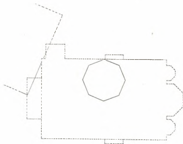
Εἰκ. 1. Σχέδιον ἐπισημανθέντων θεμελίων (συνεχεῖς γραμμαὶ) εἰς τὴν θέσιν τῆς νέας ἐκκλησίας τῆς Παναγίας (διακεκομμένοι γραμμαὶ) ἐν Παλαιᾷ Κορίνθῳ.
