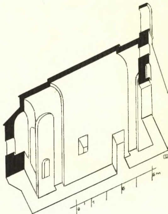
Εἰκ. 9. Τομὴ ἰσομετρικὴ τοῦ ναΐκου τῆς Παναγίας.
