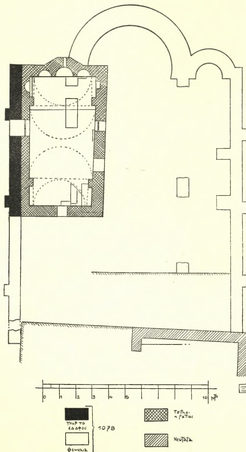
Εἰκ. 1. Κάτοψις τῶν θεμελίων τῆς βυζαντινῆς βασιλικῆς καὶ τοῦ ἐπ' αὐτῶν ναύσκου τῆς Παναγίας.
