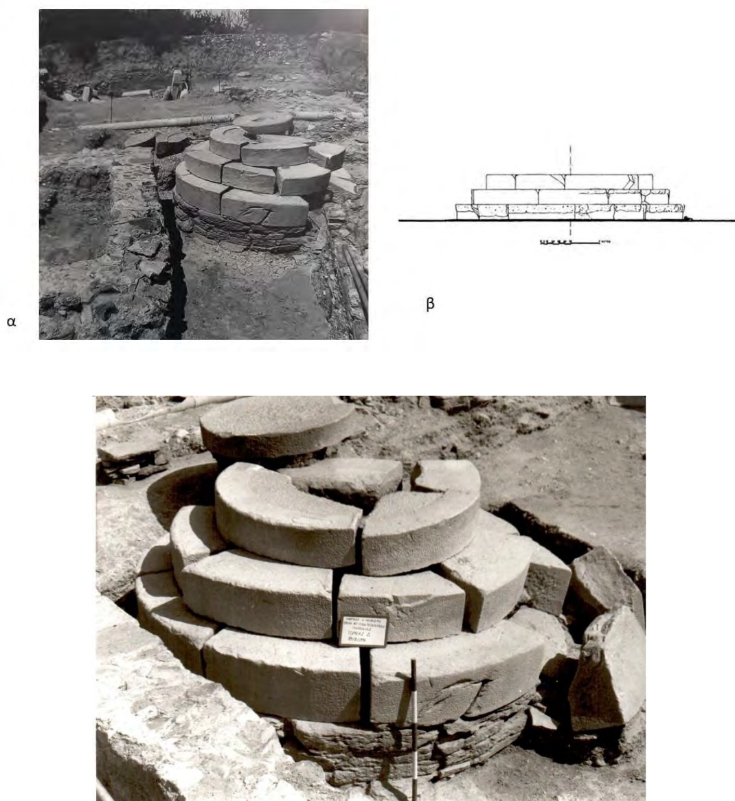
Εικ. 31, α) Το κυκλικό μνημείο στην Πάρο στη θέση Αγ. Παντελεήμων (Zaphiropoulou 2000. και β) σχεδιαστική τομή του μνημείου του Θεαγένους στη Θάσο, (Salviat 1956, εικ.11), γ) Το κυκλικό μνημείο πριν την αναστήλωσή του (αρχείο ΕΦΑ ΚΥΚΛΑΔΩΝ)
