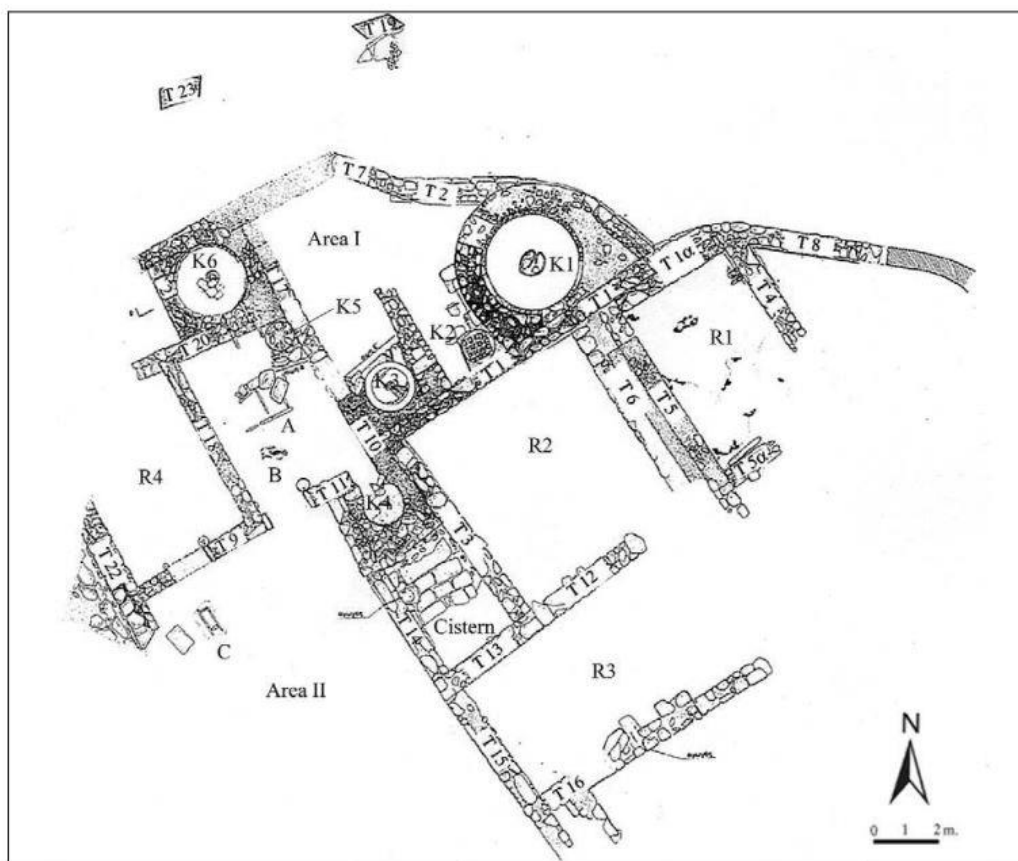
Εικ.129, Οικόπεδο Σκιαδά, Θέση Θόλος. Κάτοψη του χώρου των εργαστηρίων (Hasaki-Kouragos ΑΔ, 2012-2013)
