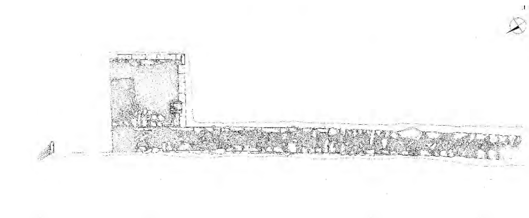
Εικ.9, Οικόπεδο Κ. Ακάλεστου, Θέση «Δύο πλάκες». Κάτοψη του τείχους στο και του πύργου (αρχείο ΕΦΑ Κυκλάδων)
