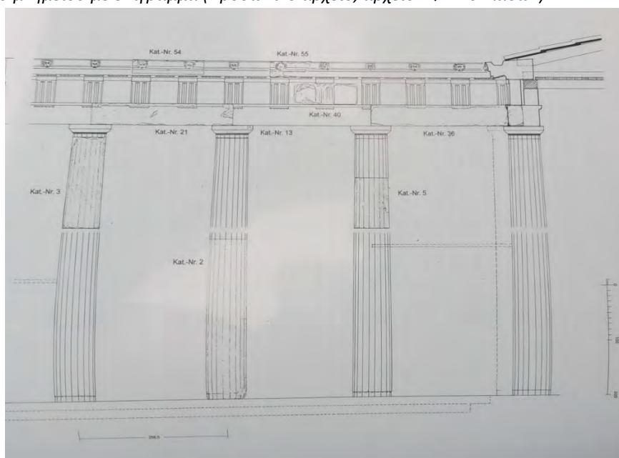
Εικ. 108, Σχεδιαστική αποκατάσταση όψης της στοάς της αγοράς της Πάρου (Muller 2003, 50, εικ.19)
