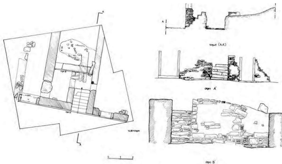
Εικ.119, Οικόπεδο Γ. Μαούνη, θέση «Φλόγα» Αριστερά κάτοψη της οικίας και Δεξιά: Τομή ΑΑ και όψεις (ΑΔ -1987- Β2, σχ.6, 497).
