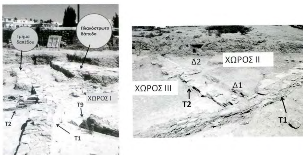
Εικ.137, Οικόπεδο Ε. Σαρρή, θέση Θόλος. α. Ο ΤΧ 1 και Βόρεια και ανατολικά του το πλακόστρωτο δάπεδο και ο πρωϊμότερος ΤΧ9. ΒΔ του ο Χώρος 2 και το δάπεδο χρήσης του ΤΧ1. β. Ο ΤΧ2 και κάθετος στον ΤΧ 1, που διαιρεί τη προς δυτικά του ΤΧ 1 έκταση σε Χώρο I και Χώρο II. Ο Χώρος II διαιρείται σε δυο δωμάτια Δ1 και Δ2 και το Δ2 έχει πήλινο αγωγό. (Παπαδημητρίου 2018)
