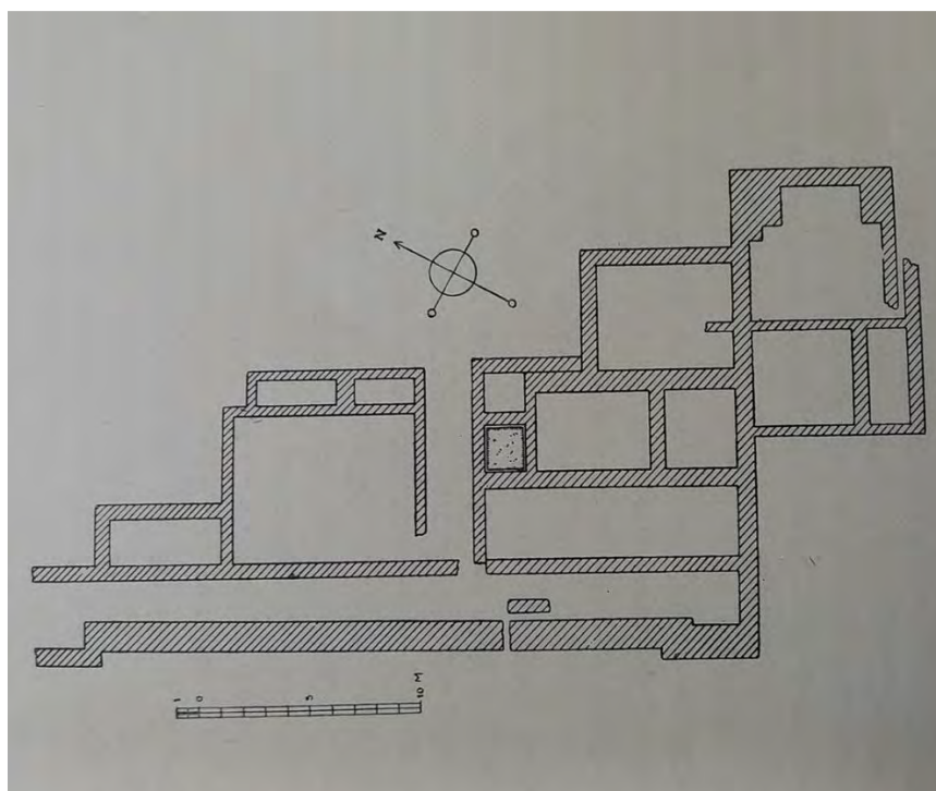
Εικ.122, Σχέδιο του Rubensohn του οικοδομήματος στη θέση Λειβάδια, (Rubensohn 1901,191)
