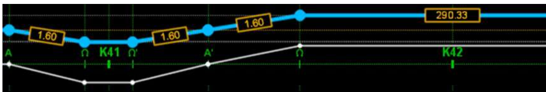
Εικόνα 34: Διορθωμένο Διάγραμμα Υπερυψώσεων
