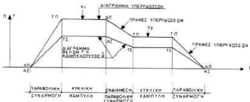
Σχήμα 2-6: Διάγραμμα Καμπυλότητας και Υπερυψώσεων Ομόστροφων Διαδοχικών Καμπυλών (N.K.E.Γ. 2000)
