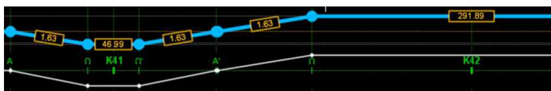
Εικόνα 31: Διάγραμμα Υπερυψώσεων
