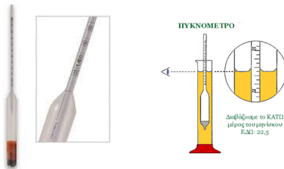
Σχήμα 2.4 Πυκνόμετρο και πως γίνεται η σωστή ανάγνωση ένδειξης (Σεϊντάνης, 2011)
