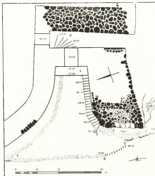
Εἰκ. 1. Ὁ μυκηναϊκὸς πύργος τῆς Ἀκροπόλεως. Σχέδιον Σ. Ἰακωβίδου.
