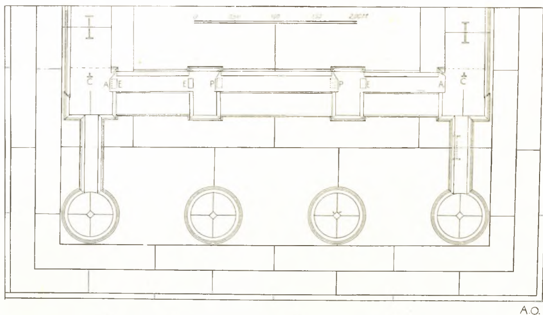
Εἰκ. 25. Πρόναος καὶ θυρώματα τοῦ ναοῦ τῆς Ἀθηνᾶς Νίκης.
