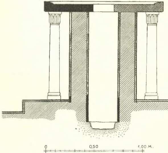
Εἰκ. 5. Τομὴ τῆς ἀγ. Τραπεζῆς τοῦ διακονικοῦ ἐν ἀναπαράστασει.
