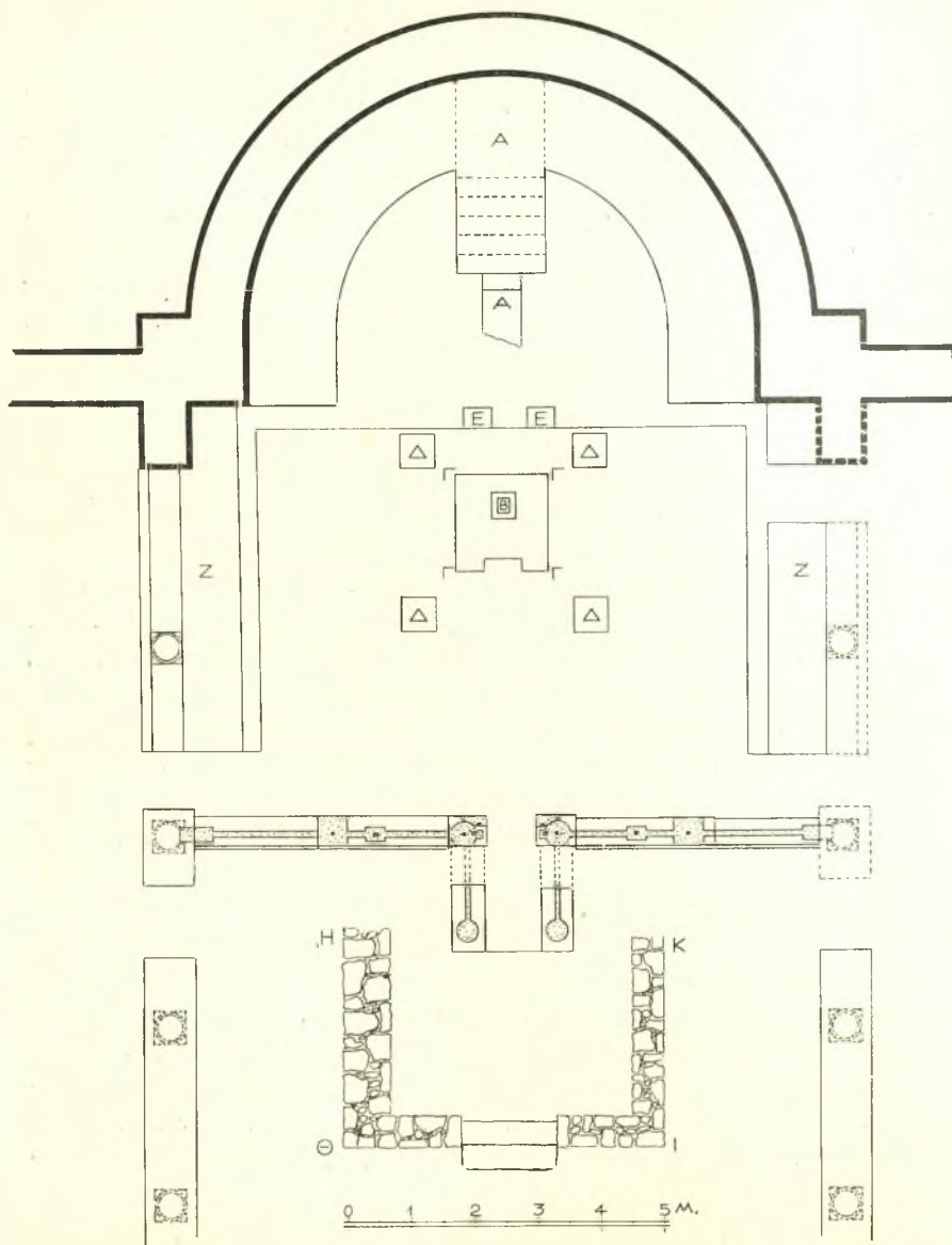
Εἰκ. 1. Κάτοψις τοῦ κυρίως ἱεροῦ καὶ τοῦ πρὸ τοῦ τέμπλου τμήματος τοῦ μέσου κλιτοῦς τῆς βασιλικῆς τῆς Σικυῶνος.
