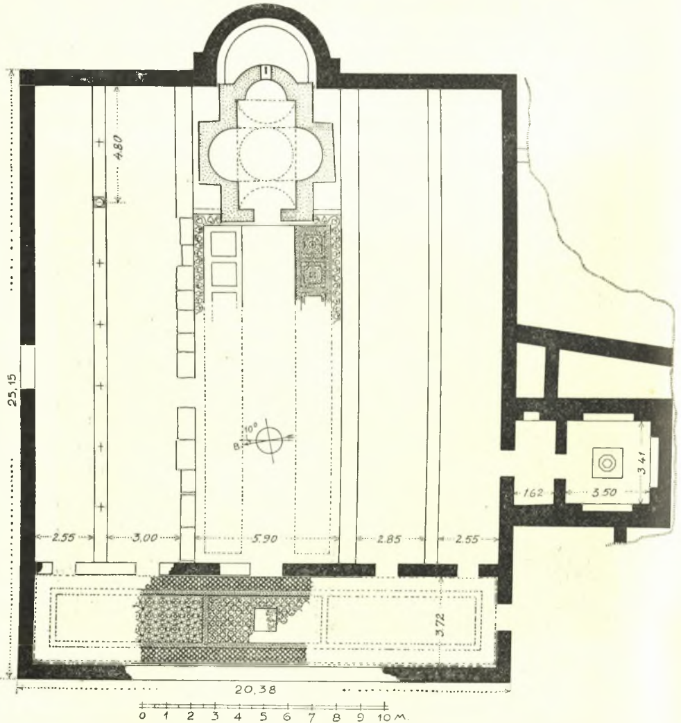
Εἰκ. 2. Κάτοψις τῆς παλαιοχριστιανικῆς βασιλικῆς τῶν Αἰγιοσθένων.
