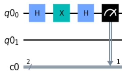
Σχήμα: 5 – Κβαντικό κύκλωμα δύο qubits
