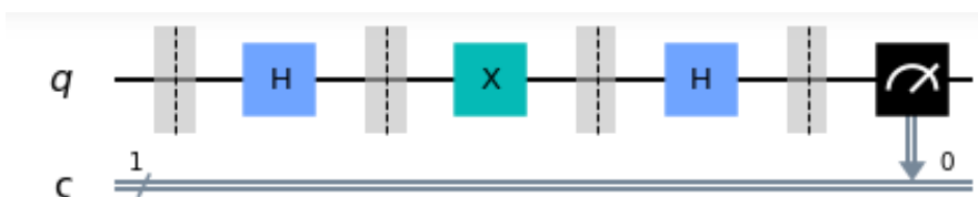
Σχήμα: 7 – 1 η Περίπτωση ο παίκτης Α δρα με πύλη X
