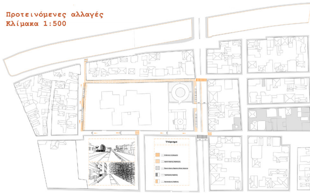
Προτεινόμενη περίφραξη του χώρου και σχεδιασμός περιβάλλοντα χώρου Κλίμακα 1:500
