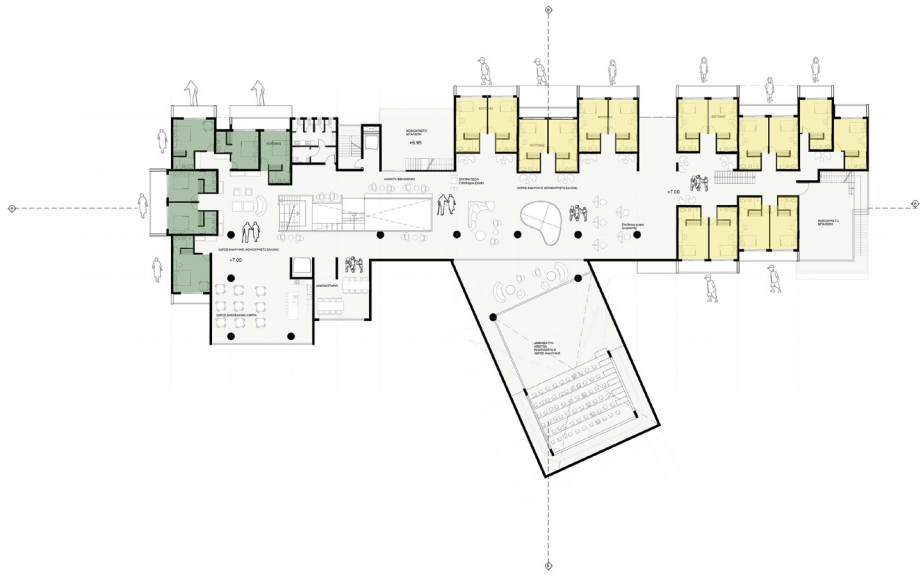
ΚΑΤΩΦΗ ΔΕΥΤΕΡΟΥ ΟΡΟΦΟΥ
