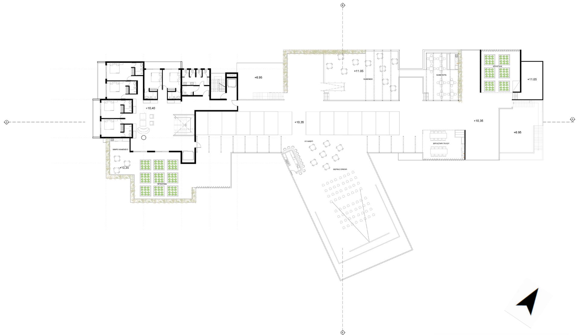
Κάτοψη τρίτου ορόφου-δώματος
