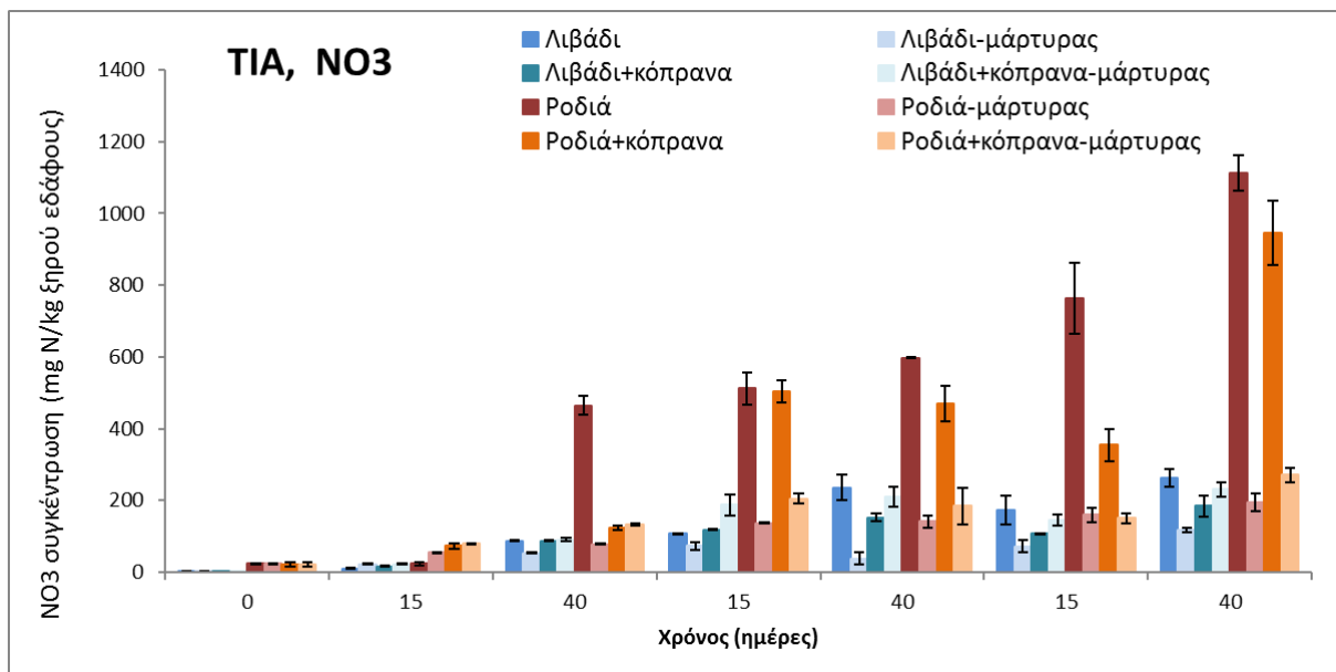
Διάγραμμα 6: Συγκέντρωση NO_3^- που προσδιορίστηκε στα δύο εδάφη, «Λιβιάδι» και «Ροδιά», στα οποία έγινε εφαρμογή TIA είτε απευθείας είτε μέσω κοπράνων σε σύγκριση με τους μεθοδολογικούς μάρτυρες, στα χρονικά σημεία 0, 15 και 40 κάθε πειραματικού κύκλου. Τα δεδομένα που παρουσιάζονται εδώ είναι οι μέσες τιμές τριών επαναλήψεων με τις τυπικές αποκλίσεις.
