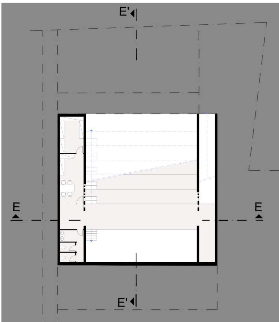
ΚΑΤΟΨΗ ΥΠΟΓΕΙΟΥ
