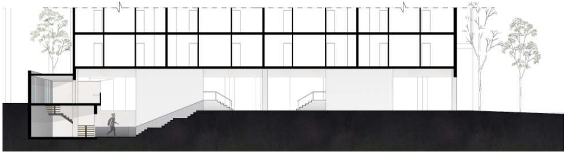
ΤΟΜΗ Β' Β'
