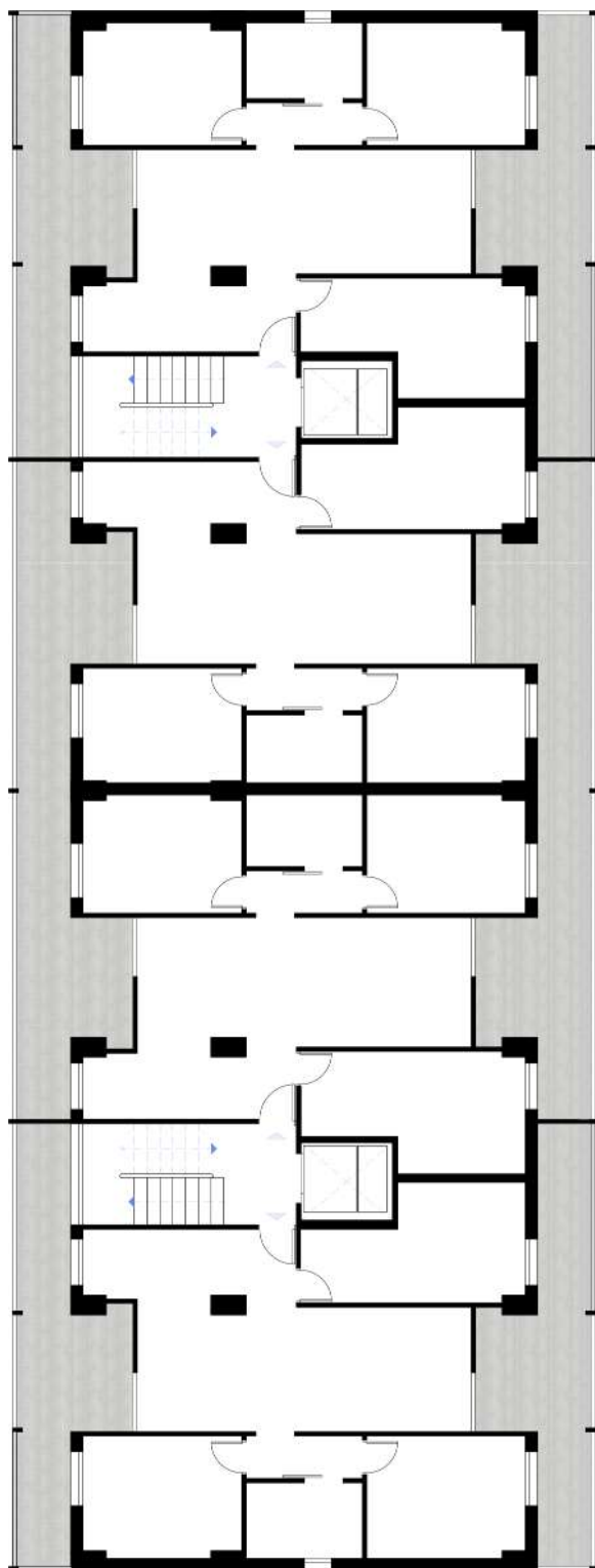
ΚΑΤΩΦΗ ΟΡΟΦΟΥ ΠΟΛΥΚΑΤΟΙΚΙΑ Α
