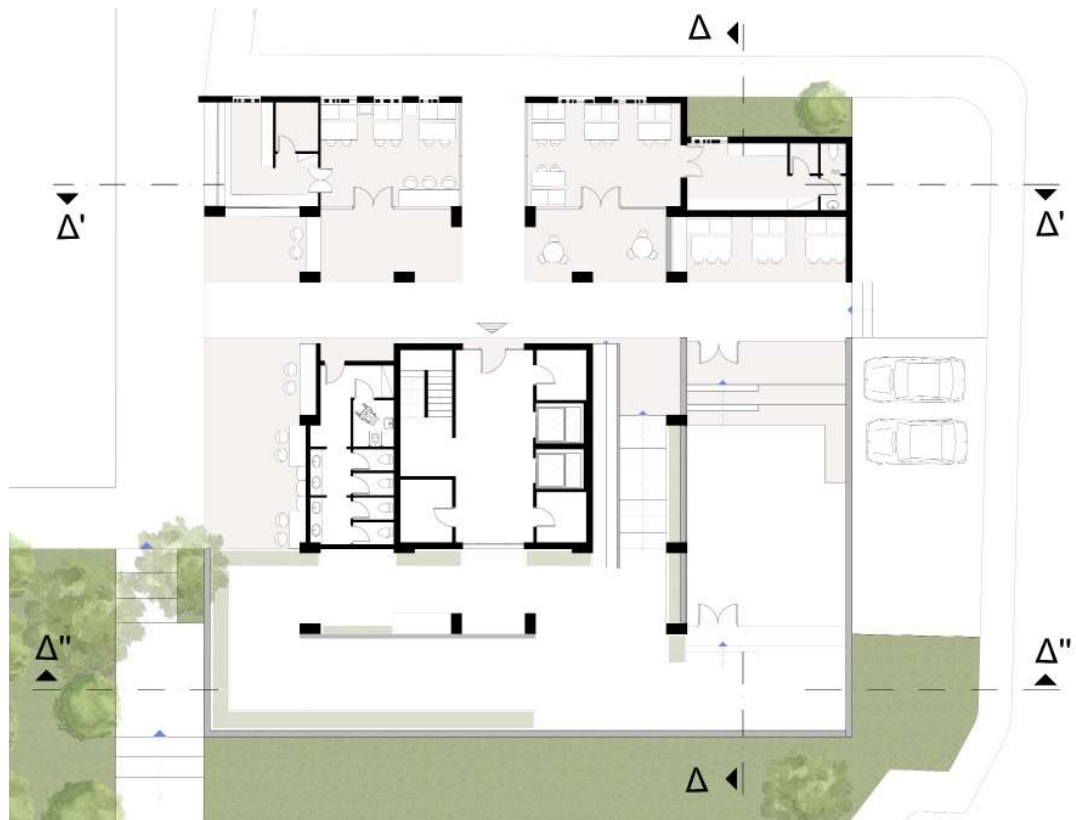
ΚΑΤΟΨΗ ΙΣΟΓΕΙΟΥ
