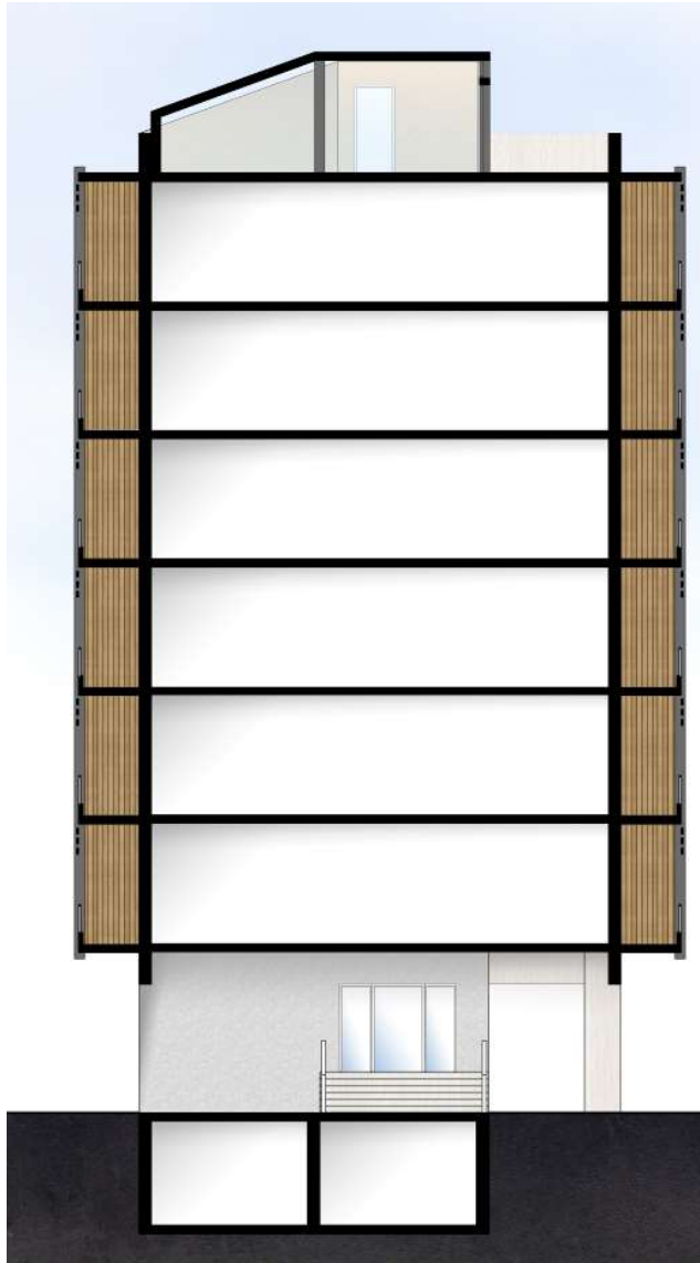
ΤΟΜΗ
