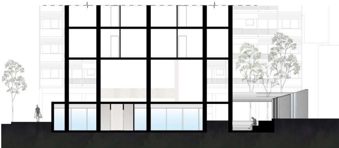
ΤΟΜΗ Γ' Γ'
