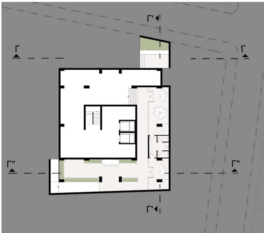
ΚΑΤΟΨΗ ΥΠΟΓΕΙΟΥ
