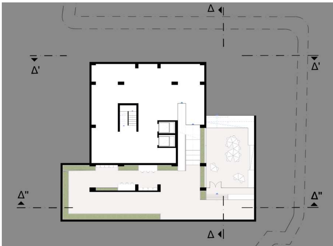
ΚΑΤΟΨΗ ΥΠΟΓΕΙΟΥ
