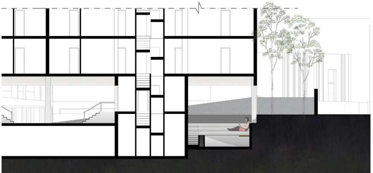
ΤΟΜΗ Β' Β'
