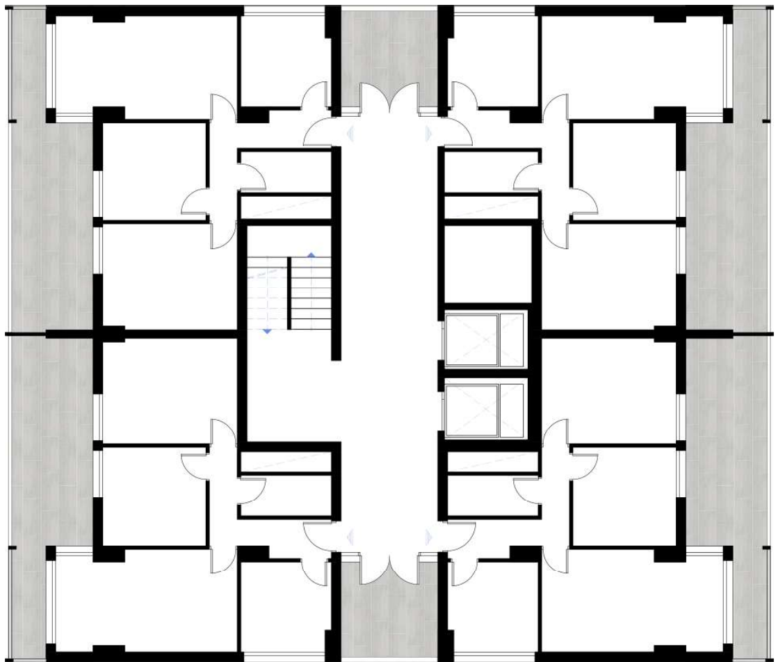
ΚΑΤΩΗ ΟΡΟΦΟΥ ΠΟΛΥΚΑΤΟΙΚΙΑ Β
