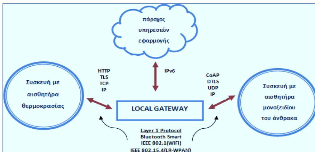
Εικόνα 11: Παράδειγμα μοντέλου επικοινωνίας Device-to-Gateway
