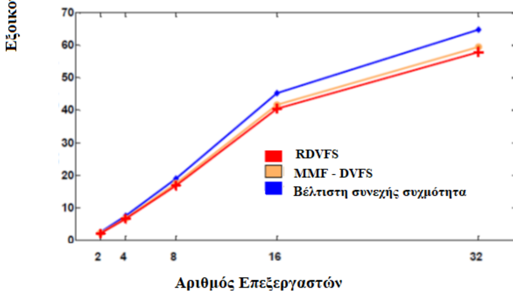
Σχήμα 3-8. Η εξάρτηση της εξοικονόμησης ενέργειας σε MMF-DVFS και άλλους αλγορίθμους στον αριθμό των επεξεργαστών: (α) 1500 τυχαία παραγόμενα γραφικά εργασίας, (β) γραφικές παραστάσεις εργασιών αποικοδόμησης 300 LU.
