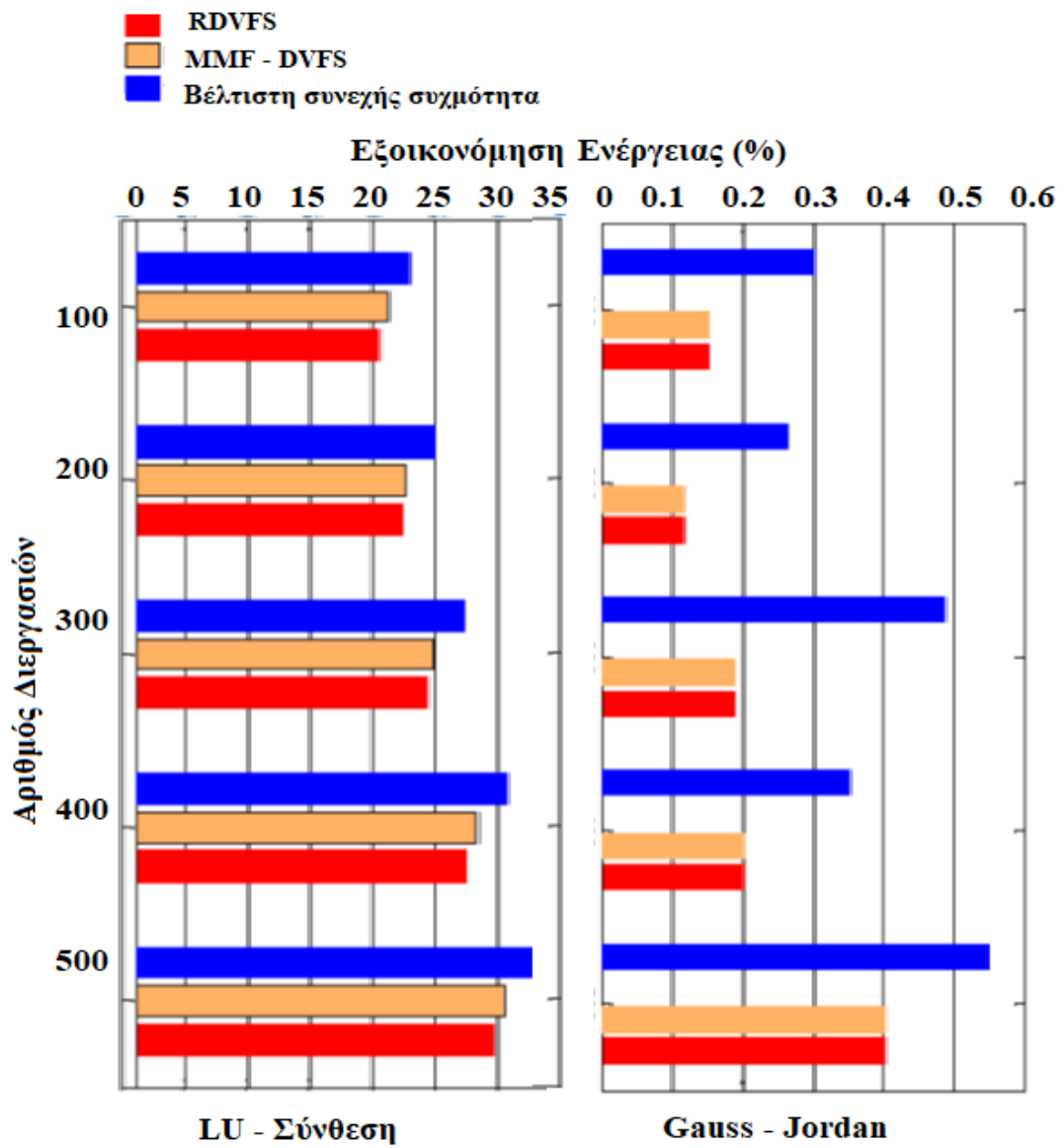
Σχήμα 3-6. Η κανονικοποιημένη κατανάλωση ενέργειας του MMF-DVFS και άλλων αλγορίθμων για τον αριθμό των εργασιών για δύο εφαρμογές πραγματικού κόσμου: σύνθεση LU, και Gauss-Jordan.
