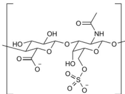
Εικόνα 2: Χημική δομή θεικής χονδροΐτινης x .
