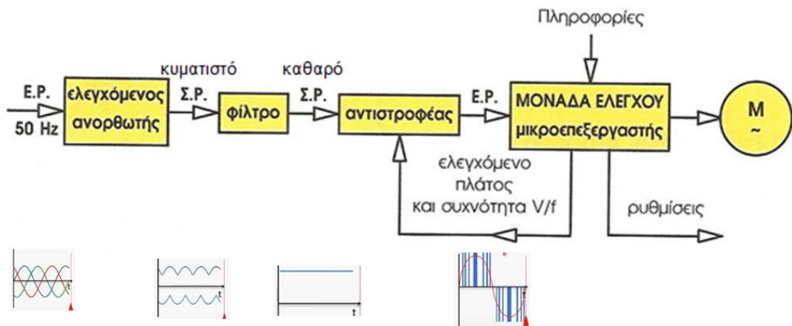
Εικόνα 52: Μέρη inverter
