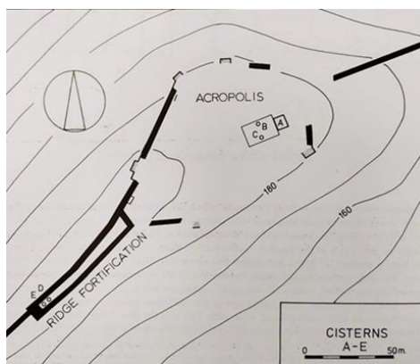
Εικόνα 2.1.3 - Λόφος Γορίτσας. Η ακρόπολη και η οχυρωμένη κορυφογραμμή με σημειωμένα τα σημεία όπου έχουν βρεθεί οι δεξαμενές (Bakhuizen 1992, εικ. 100A).
