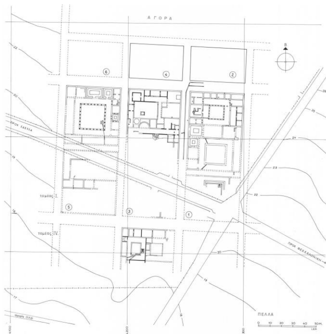
Εικόνα 4.10 – Τοπογραφικό διάγραμμα Πέλλας. Κάτοψη (αριστερά) της «Οικίας της αρπαγής της Ελένης» και (δεξιά) της «Οικίας του Διονύσου» (Μακαρόνας και Γιούρη 1989, Τοπογραφικό 1).
