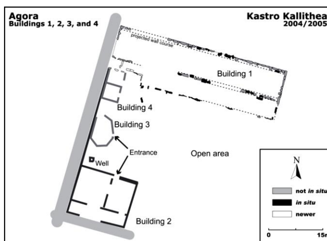
Εικόνα 3.2.7 - Κάστρο Καλλιθέας. Κάτοψη των τεσσάρων κτιρίων της αγοράς (Tzafalias et al. 2009, 227, εικ. 5).
