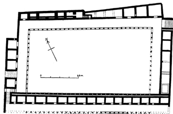
Εικόνα 4.8 – Πέργαμος. Κάτοψη της Κάτω Αγοράς (Wycheley R.E. 1942. “The Ionian Agora”. Journal of Hellenic Studies . Vol. 62: 27, εικ. 5).
