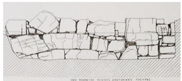
Εικόνα 1.14.3 - Κίριο. Σχέδιο της όψης του τείχους (Χατζηαγγελάκης 2000, 389, σχ. 12).
