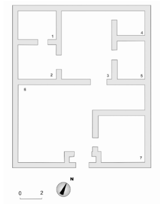
Εικόνα 3.1.9 – Άλος. Κάτοψη της «Οικίας του Αγάθωνα» (Haagsma 2010, 72, εικ. 2.41).
