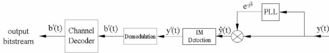
Figure 7: Ο Δέκτης/Rx του συστήματος.
