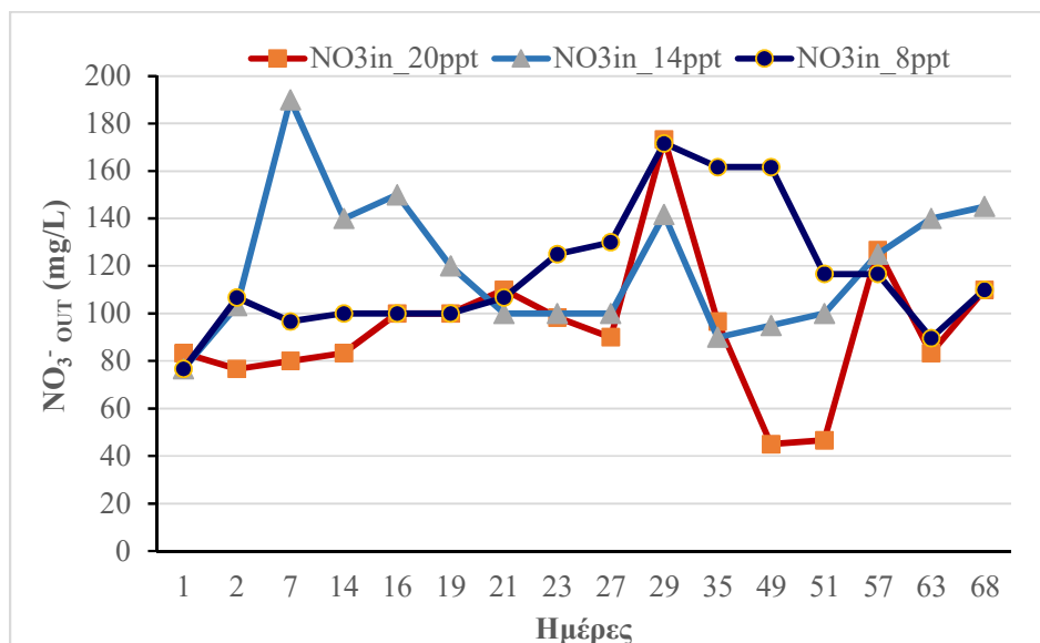
Σχήμα 4. Διάγραμμα μεταβολής των νιτρικών ιόντων ( \text{NO}_3^-_{\text{in}} ) στο σημείο εισόδου του νερού στην υδροπονική δεξαμενή καλλιέργειας του κρίταμου του ενυδρείοπονικού συστήματος με αλατότητα 8 ppt, 14 ppt και 20 ppt, αντίστοιχα.
