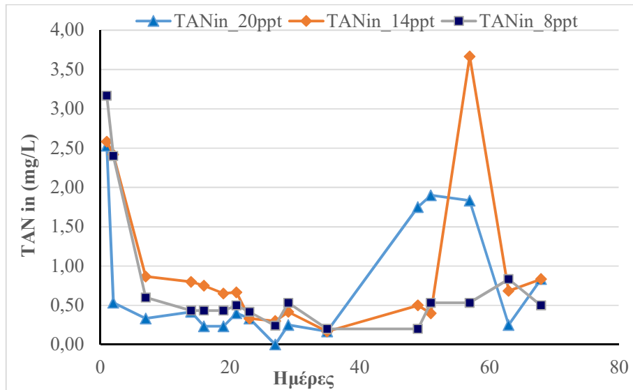
Σχήμα 1. Διάγραμμα μεταβολής της ολικής αμμωνίας ( TAN_{in} ) στο σημείο εισόδου του νερού στο φίλτρο στα ενυδρειακά συστήματα ανακυκλοφορίας νερού του ενυδρειοπονικού συστήματος με αλατότητα 8 ppt, 14 ppt και 20 ppt, αντίστοιχα.
