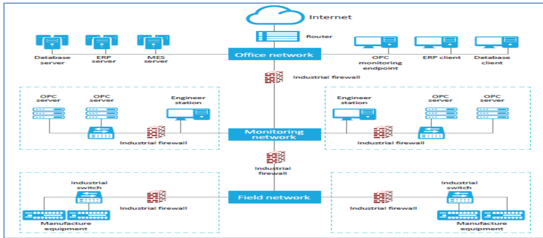
Εικόνα 20: Εφαρμογή βιομηχανικών τειχών προστασίας (Πηγή: Building a Trusted and Managed IoT World)
