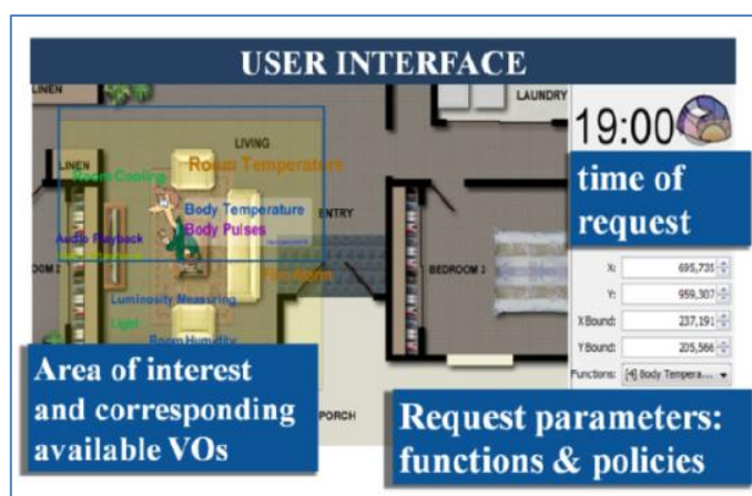
Εικόνα 8: Γραφικό περιβάλλον διεπαφής χρήστη (Πηγή: The IEEE International Conference on Internet of Things)
