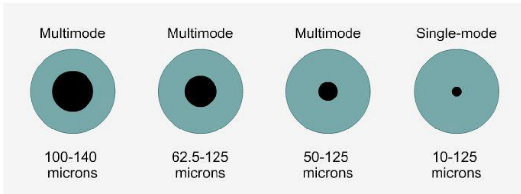
(Διάμετρος των πυρήνων multimode και singlemode ιών)
