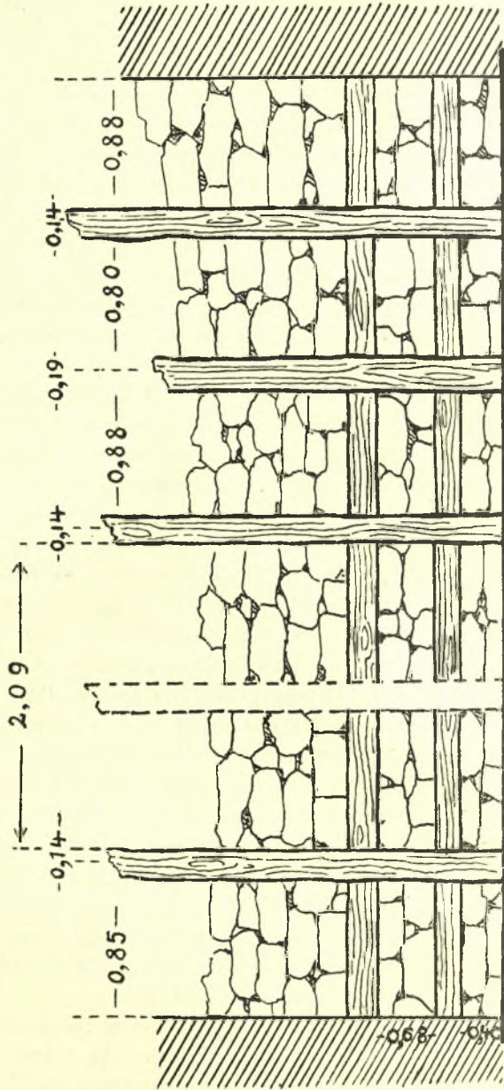
Εἰκ. 5. Σχηματικὴ ἀναπαράστασις τῆς ὄψεως τοῦ βορείου τοίχου τοῦ θαλάμου Π δεικνύουσα τὴν ξυλόδεσιν αὐτοῦ. (Οἱ λίθοι εἶνε κατὰ φαντασίαν, οὐχὶ κατ' ἀντιγραφήν. Ὑπερ τὴν ἄνω ζώνην δὲν δέκοντα ἀλλήν, ἀλλὰ πιστεύω, ὅτι ὑπέρχον καὶ ἄλλαι).
