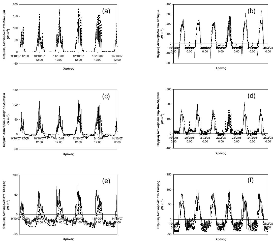
Σχήμα 6.11 (a), (b), (c), (d), (e), (f). Διακύμανση των μετρημένων (—) και υπολογισμένων (---) τιμών της καθαρής θερμικής ακτινοβολίας στο κάλυμμα, στην καλλιέργεια και στο έδαφος κατά τη διάρκεια δύο πειραματικών περιόδων.
