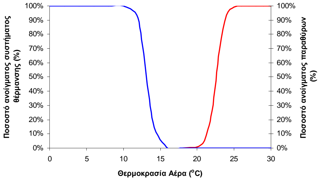
Σχήμα 11.10. Ποσοστό ανοίγματος (%) του συστήματος θέρμανσης και των παραθύρων κατά τη διάρκεια της 3 ης πειραματικής περιόδου προσομοίωσης
