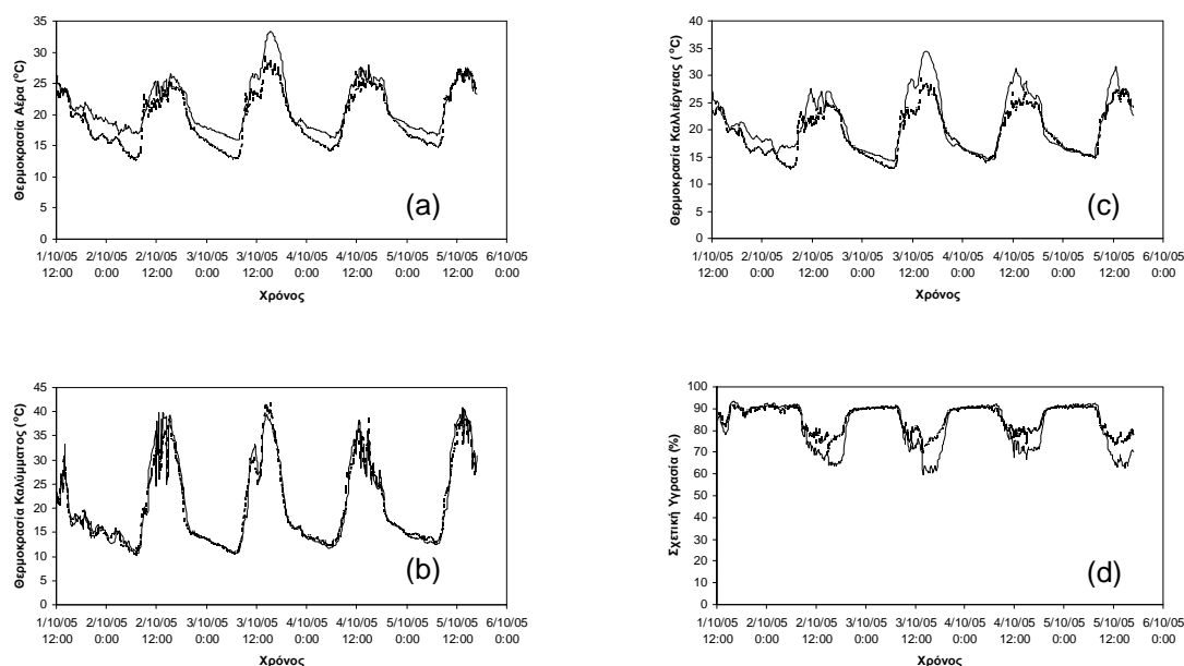
Σχήμα 6.14. (a), (b), (c), (d). Διακύμανση των μετρημένων (—) και υπολογισμένων (---) τιμών της θερμοκρασίας του αέρα, του καλύμματος της καλλιέργειας και της σχετικής υγρασίας του αέρα, για την πειραματική περίοδο 2005-2006.
