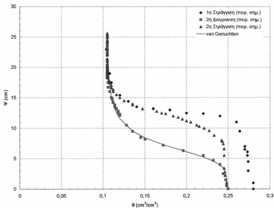
Σχήμα 4.22 Χαρακτηριστικές καμπύλες πρώτου εδαφικού δείγματος [αμμώδους (S)], για την 1 η στράγγιση, τη 2 η διύγρυνση και τη 2 η στράγγιση
