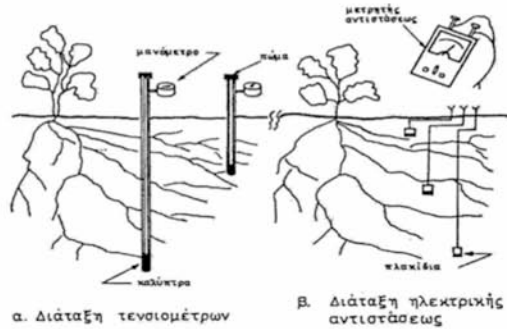
Σχήμα 3.1 Διάταξη тенσιομέτρων και πλακιδίων ηλεκτρικής αντιστάσεως για τον προσδιορισμό της τάσης της εδαφικής υγρασίας
