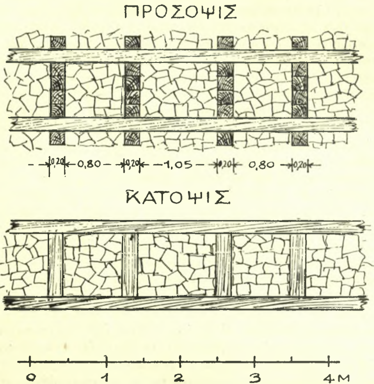
Εἰκ. 2. Πῶς φανταζόμεθα τὴν κτίσιν τοῦ βορείου τοίχου τοῦ αὐτοῦ δωματίου Ν (πρβλ. εἰκ. 1).
