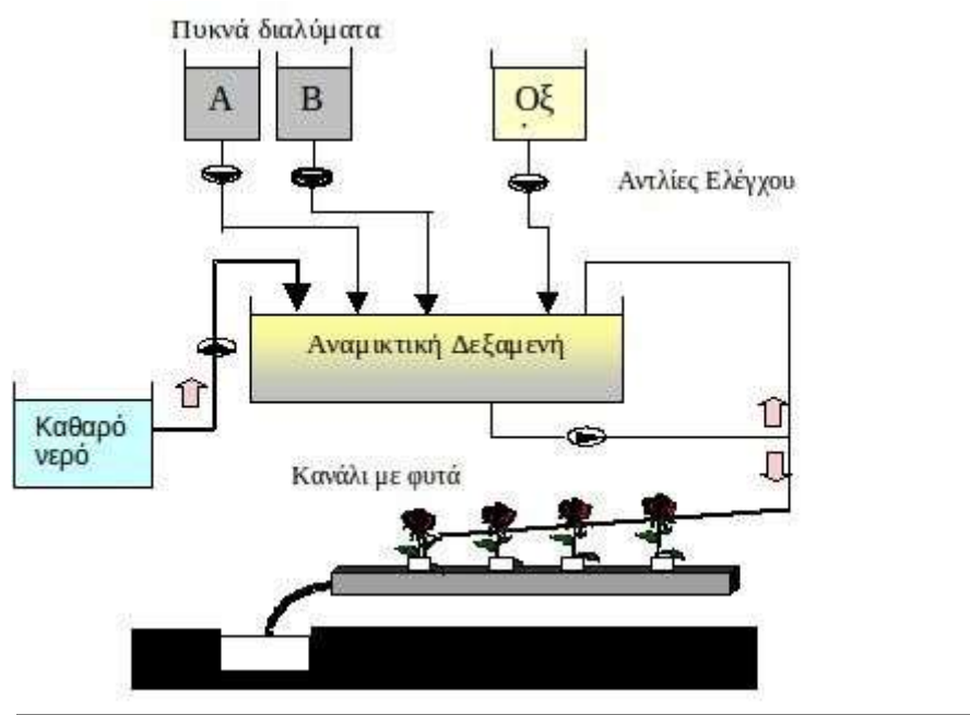
Σχεδιάγραμμα 1. σχεδιάγραμμα ανοικτού (χωρίς ανακύκλωση) υδροπονικού συστήματος Α/Β δεξαμενών με χρήση αναμικτικής δεξαμενής. (Πηγή: http://www.alagro.gr/en/anoixta-systhmata/ )
