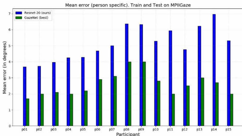
Σχήμα 5.2: Εκπαίδευση και αξιολόγηση μοντέλων με δεδομένα από το ίδιο άτομο της βάσης MPIIGaze (person-specific evaluation). Οι τιμές εκφράζουν το μέσο σφάλμα καθενός από τους 15 συμμετέχοντες του MPIIGaze.
