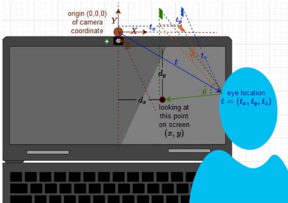
Σχήμα 4.1: Παράδειγμα ανίχνευσης σημείου στην οθόνη με δεδομένο το διάνυσμα μετατόπισης t , τις γωνίες βλέμματος \hat{\phi} , \hat{\theta} και ζητούμενο το σημείο (x, y) της οθόνης.
