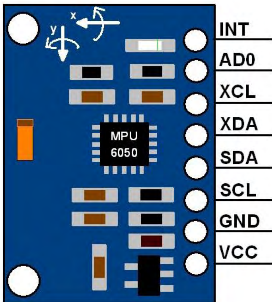
Εικόνα 16: MPU-6050.
