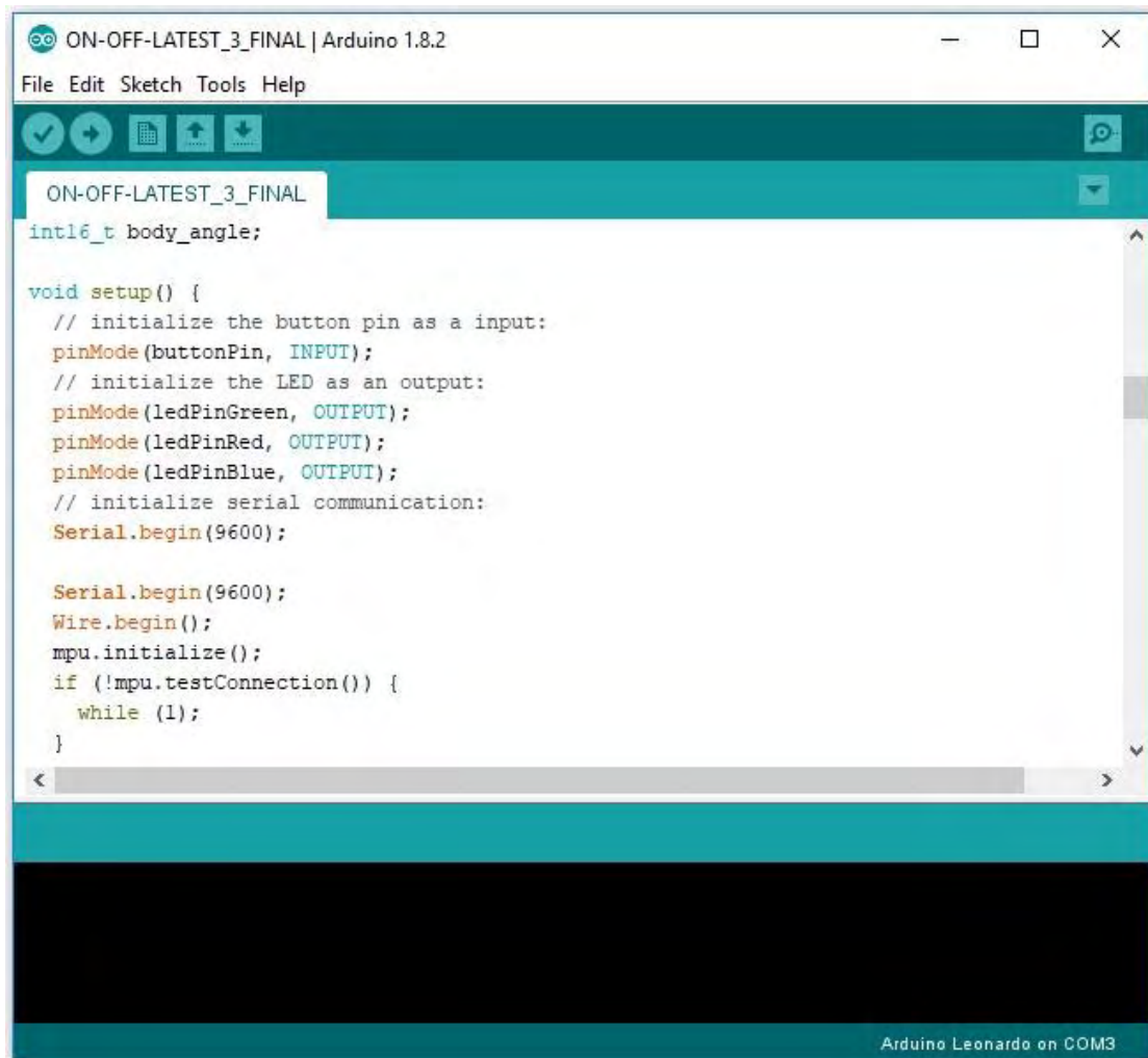
Εικόνα 15: Arduino IDE.
