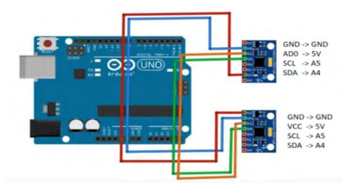
Εικόνα 24: Σύνδεση Arduino με 2 MPU-6050.
