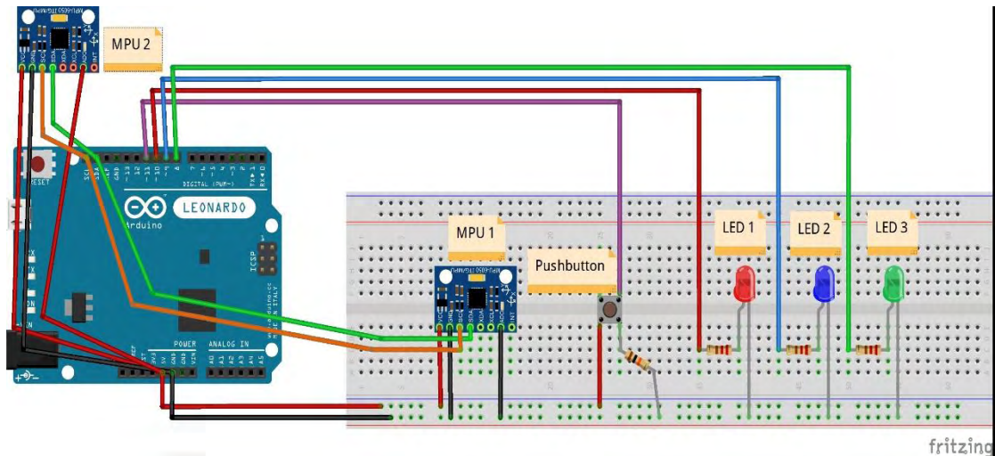
Εικόνα 25: Ολοκληρωμένη κατασκευή τελικού συστήματος Arduino Leonardo με 2 MPU-6050.
