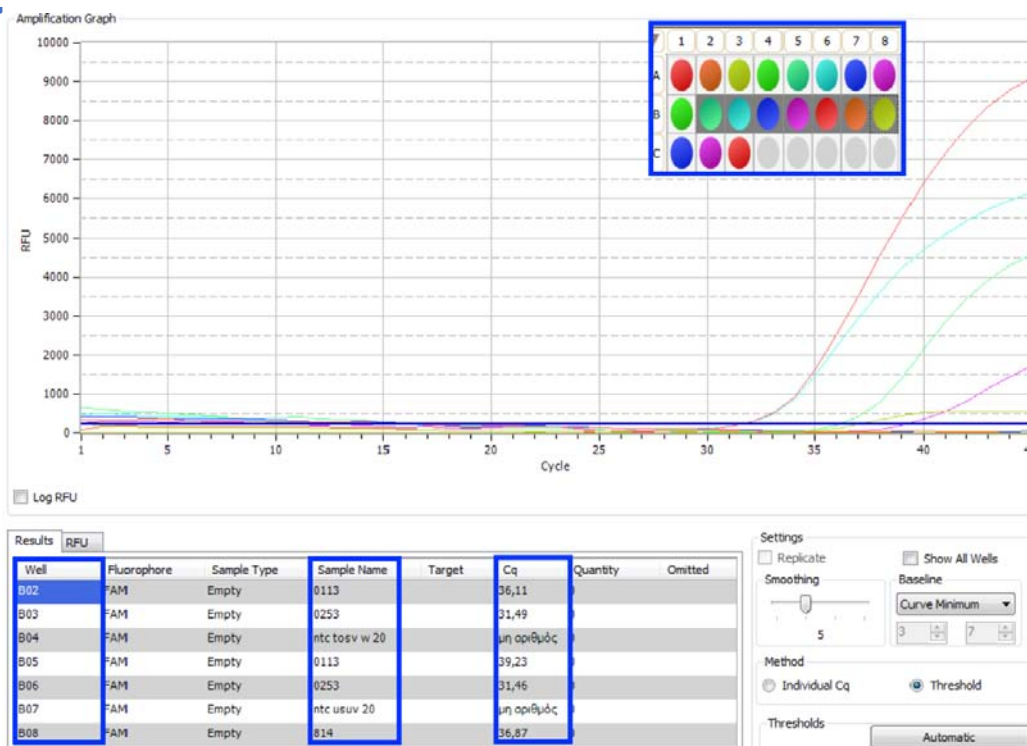
Εικόνα 13: Καμπύλες πολλαπλασιασμού των θετικών μαρτύρων «814» (USUV +) και «0253» (TOSV +) με χρήση του κιτ PCR BIO Probe 1-Step Go NO-Rox, της εταιρίας PCR Biosystems (Cat. No. PB25.43-03), στο μηχάνημα PikoReal24 (Thermo scientific) και με τελικό όγκο αντίδρασης 20 µl.
