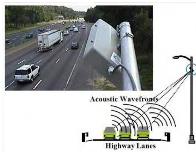
Σχήμα 3- 7: Ακουστικός αισθητήρας για καταμέτρηση οχημάτων
