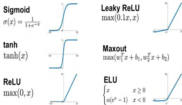
Σχήμα 5- 5: Συναρτήσεις ενεργοποίησης
