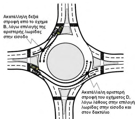
Σχήμα 3.3-3: Συγκρούσεις κατά την έξοδο λόγω λάθους στην επιλογή λωρίδας από την έναρξη της εισόδου στο δακτύλιο (Πηγή: ΟΜΟΕ – Κ3)
