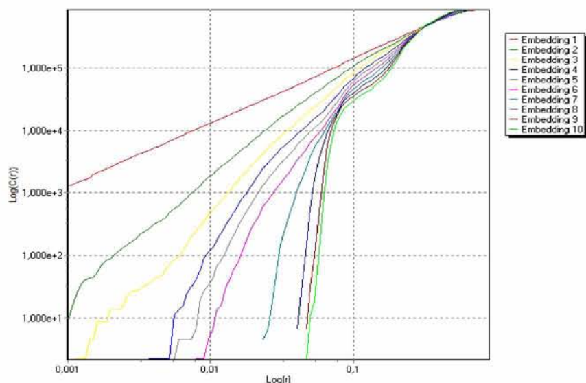
Εικόνα 2.6. Αριθμός σημείων που συμπεριλαμβάνονται σε κάθε διάσταση στον μετασχηματισμένο ελκυστή
