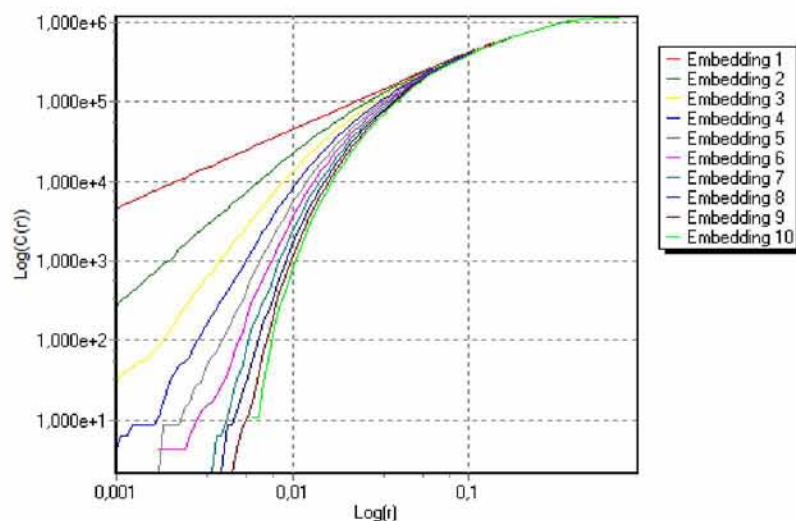
Εικόνα 2.15. Αριθμός σημείων που συμπεριλαμβάνονται σε κάθε διάσταση στον μετασχηματισμένο ελκυστή
