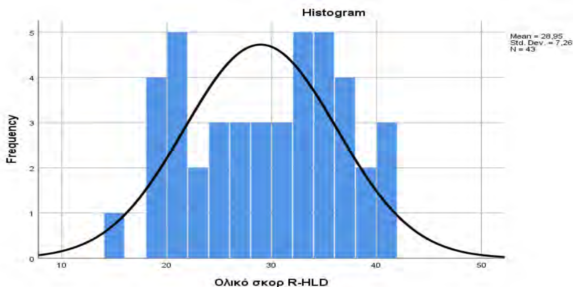
Πίνακας 5: Απόδοση ολικής βαθμολογίας R-HLD στο δείγμα
