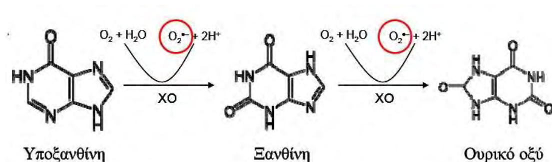
Εικόνα 5: Δράση της οξειδάσης της ξανθίνης και παραγωγή ρίζας σουπεροξειδικού ανιόντος.
