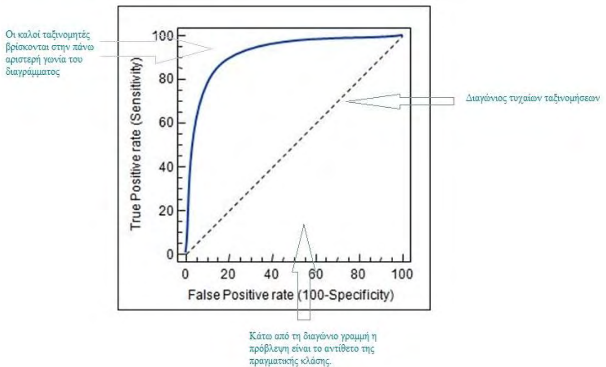
Εικόνα 27: Καμπύλη ROC
