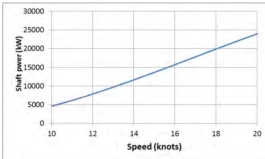
Διάγραμμα 5. Διάγραμμα ισχύος άξονα-συναρτήσεϊ ταχύτητας GPS πλοίου για τα πλοία 137 & 45 για ταχύτητα από 10 έως 20 knots με βάση την πολυωνομική εξίσωση.
