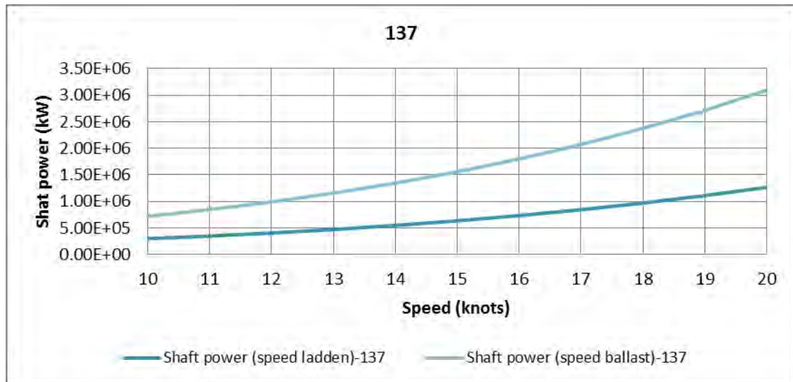
Διάγραμμα 3. Σύγκριση καμπυλών ταχύτητας πλοίου-ισχύος άξονα στην περίπτωση φορτίου και στην περίπτωση έρματος, για το πλοίο 137.
