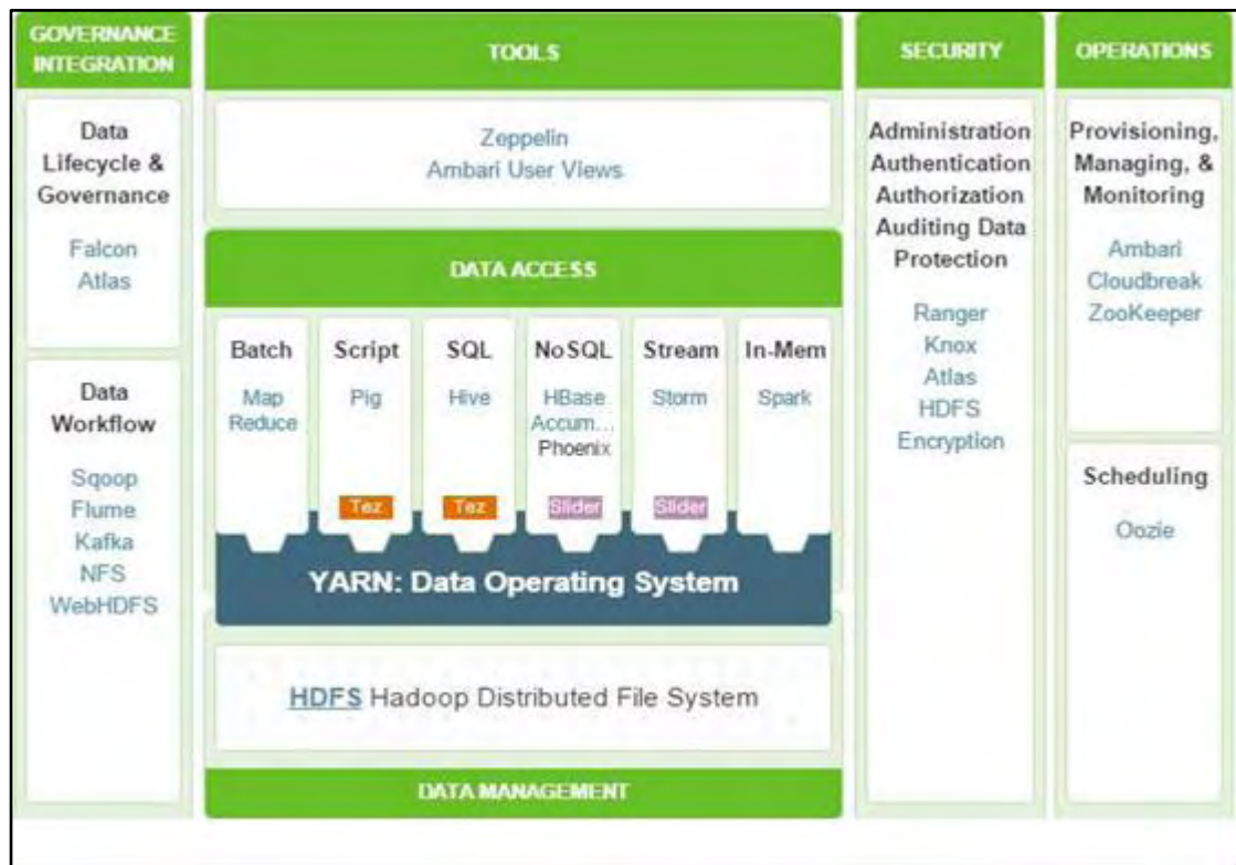
Εικόνα 10 : Οικοσύστημα Hadoop
