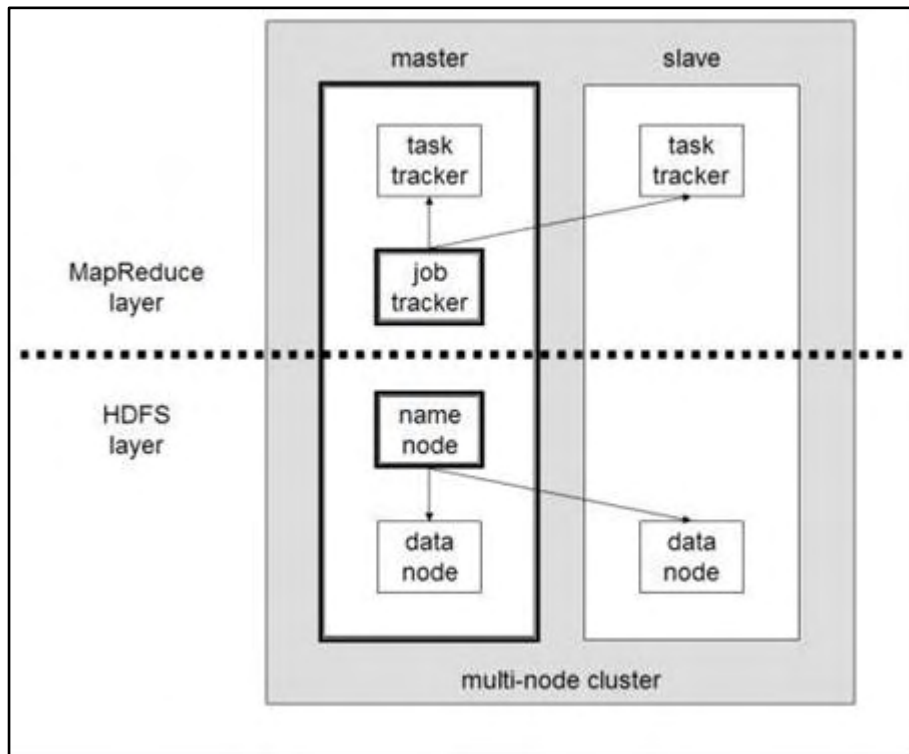
Εικόνα 4: Αρχιτεκτονική Hadoop
