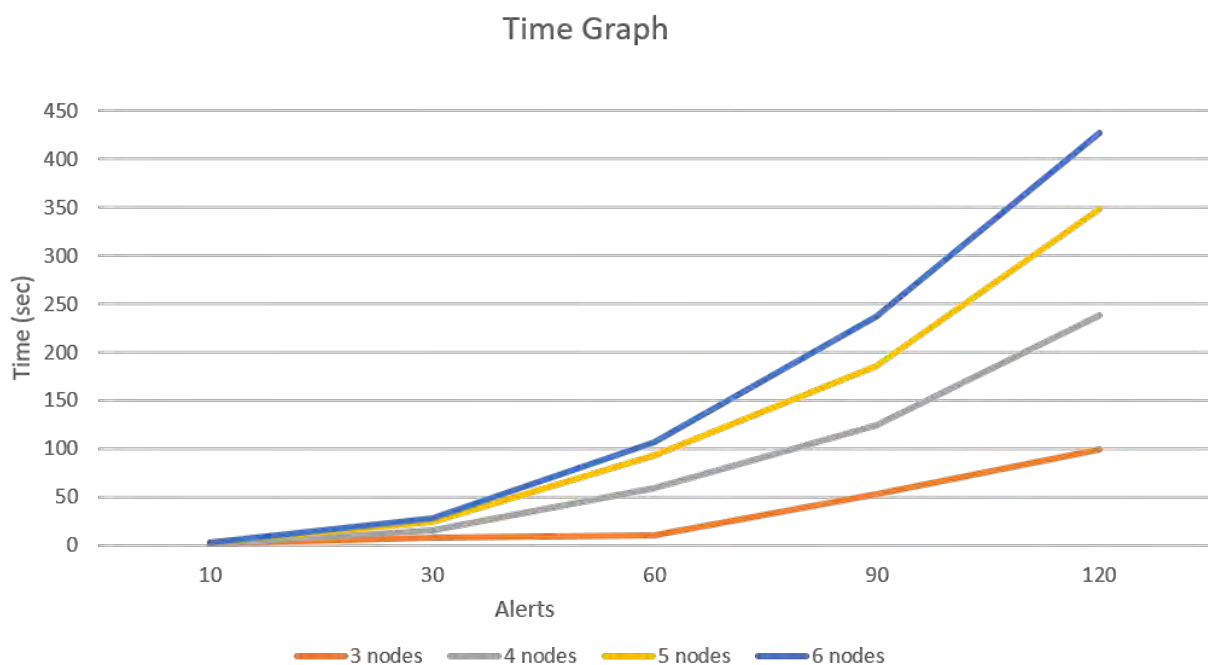
Σχήμα 5.1: Γράφημα Χρόνου εκτέλεσης
