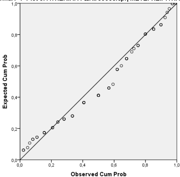
Γράφημα 50. Συμμετρίας (P-P plot) της μεταβλητής «οβελιαία αυχενική ευθυγράμμιση» την ημέρα εξόδου
