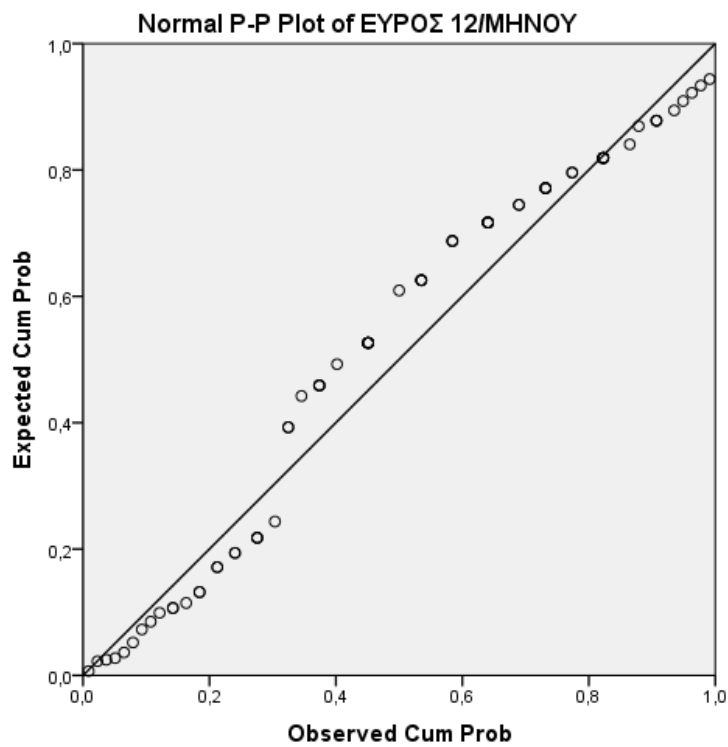
Γράφημα 57. Συμμετρίας (P-P plot) της μεταβλητής «εύρος κίνησης Α.Μ.Σ.Σ.» στο 12/μηνο
