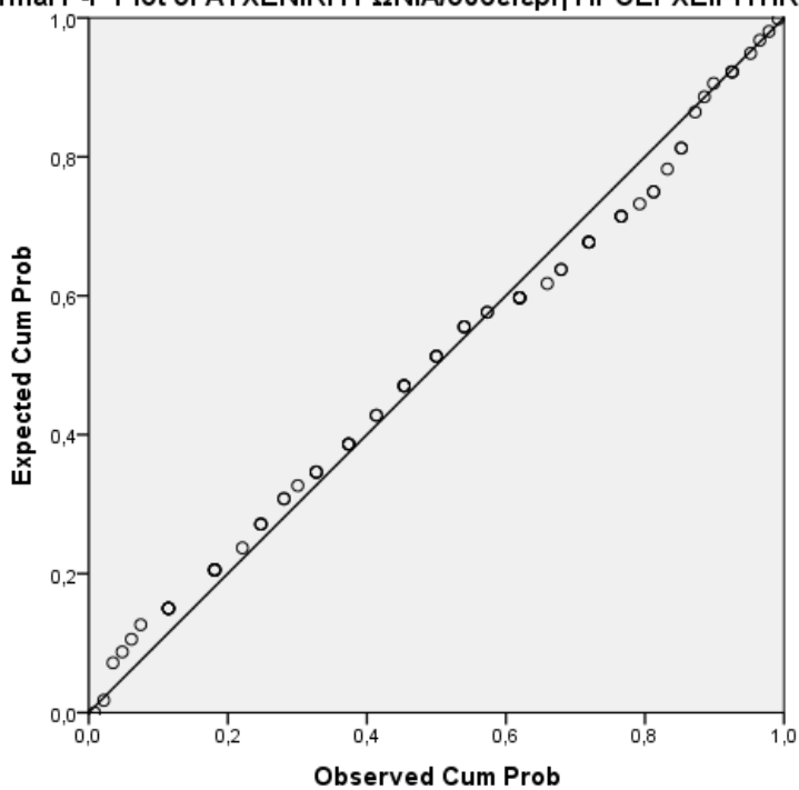
Γράφημα 49. Συμμετρίας (P-P plot) της μεταβλητής «οβελιαία αυχενική ευθυγράμμιση» προεγχειρητικά
