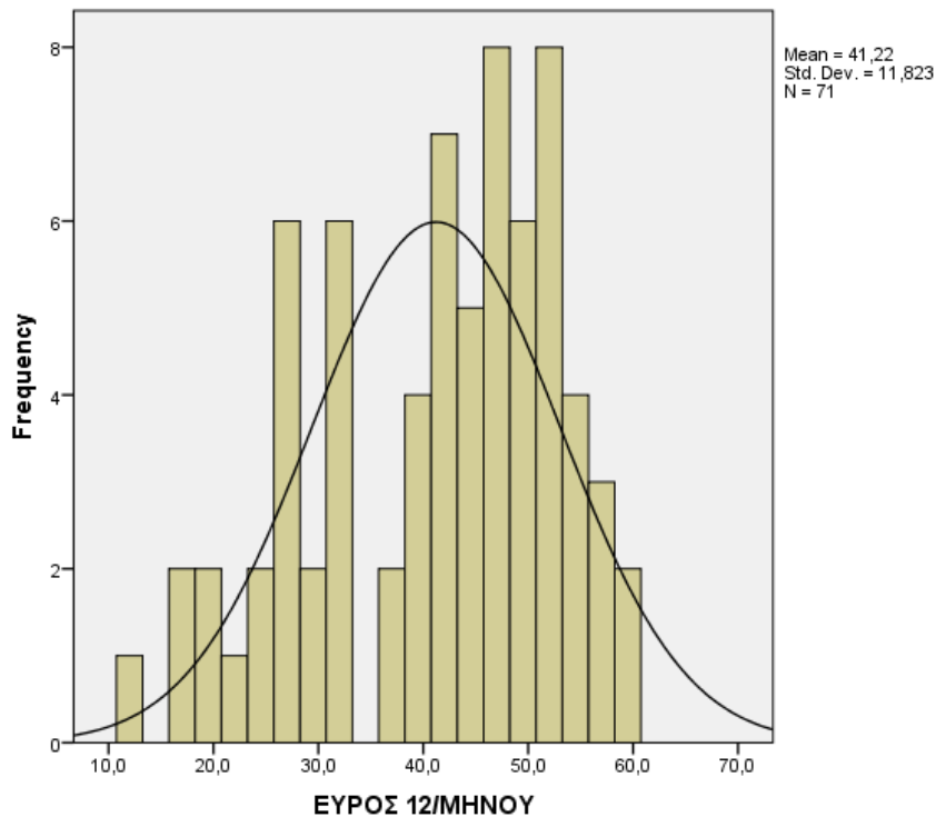
Γράφημα 54. Ιστογράμμα κατανομής συχνοτήτων της μεταβλητής «εύρος κίνησης Α.Μ.Σ.Σ.» στο 12/μηνο
