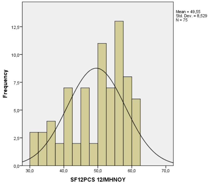
Γράφημα 35. Ιστογράμμο κατανομής συχνοτήτων της μεταβλητής «SF-12 PCS» στο 12/μηνο
